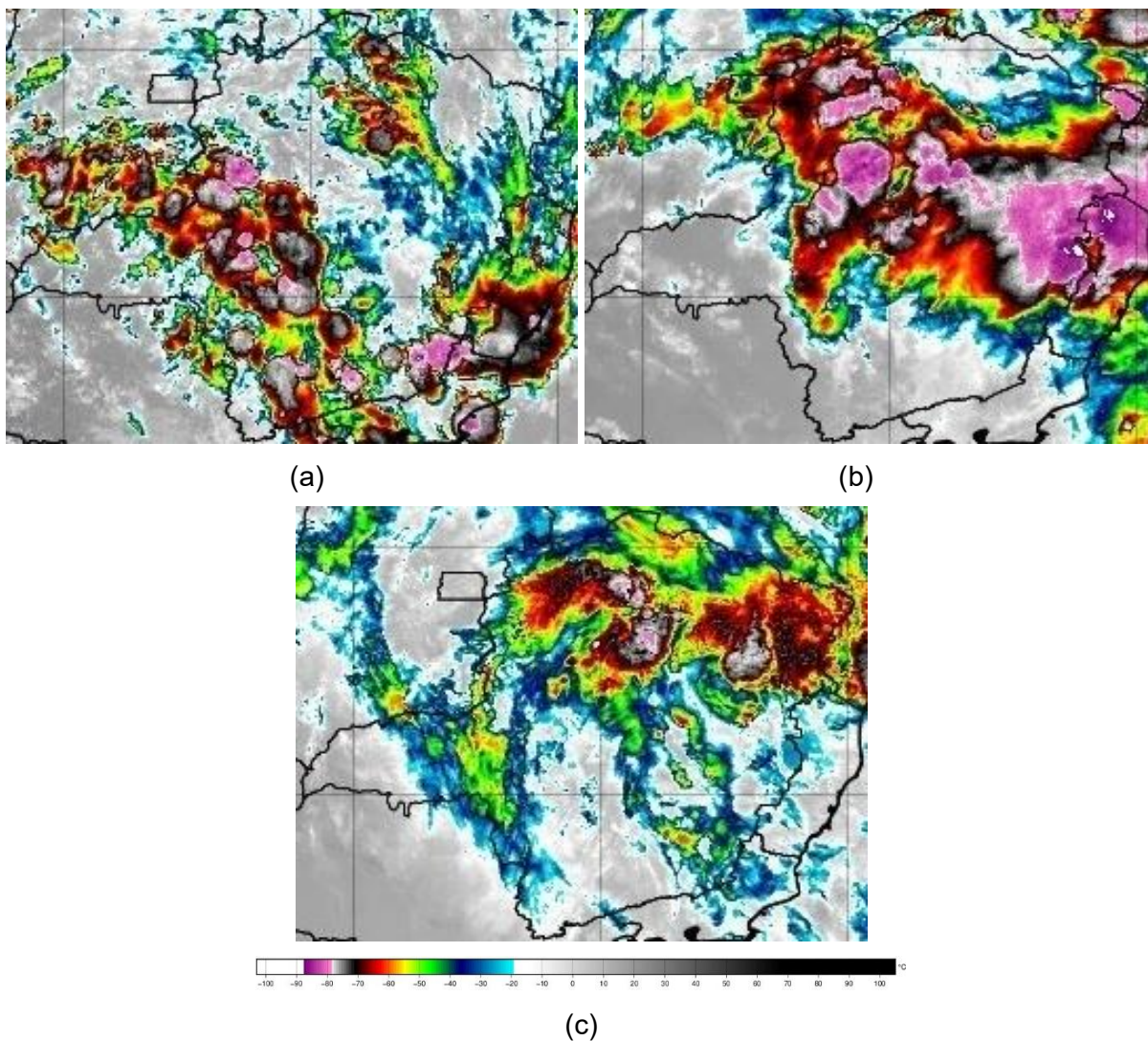
Figura 2 – Seleção de Imagem de Satélite dos dias 26 (a), 27 (b) e 28 (c) de fevereiro de 2026. Fonte: INPE.
