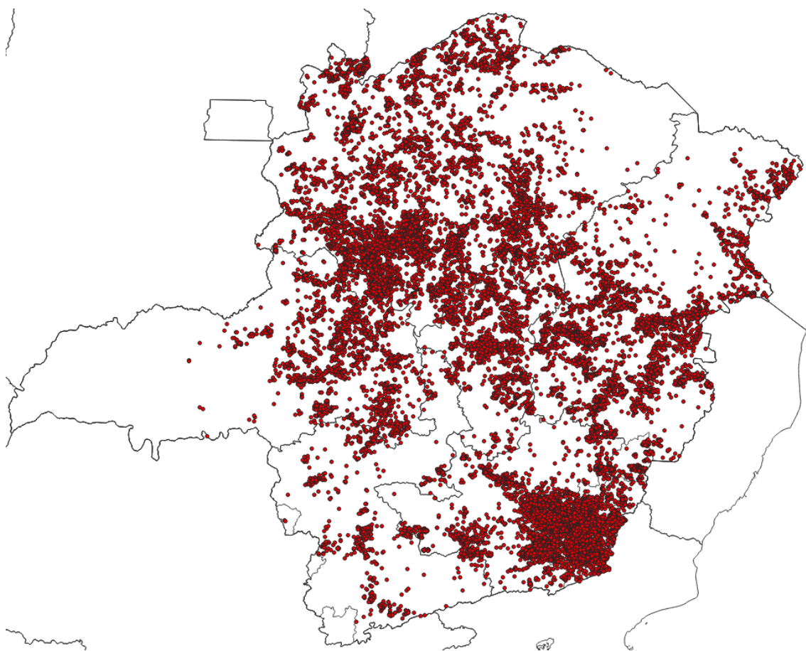
Figura 3 - Localização dos raios registrados entre os dias 26 e 28 de fevereiro de 2026. Fonte: RINDAT
