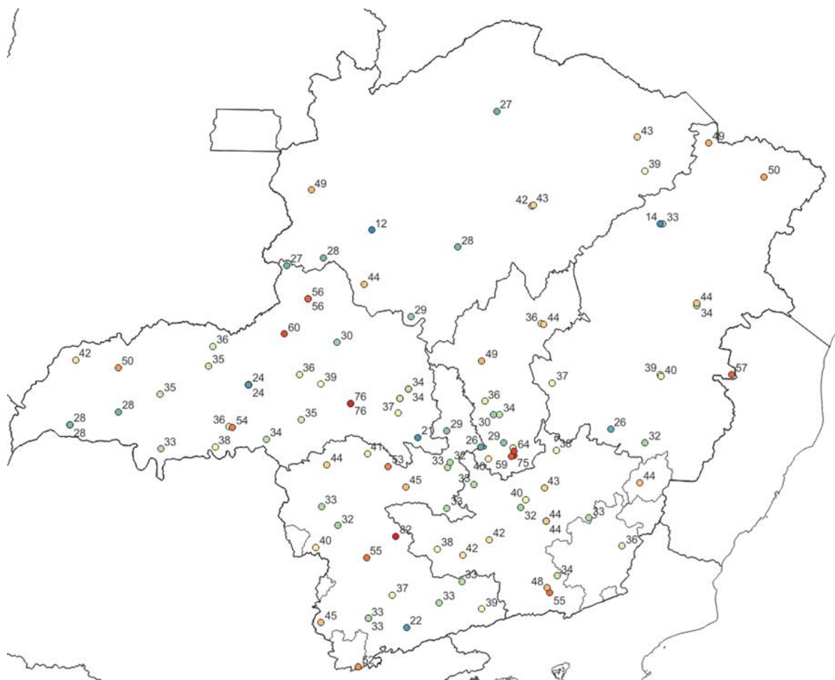
Figura 4 – Rajadas de vento (Km/h) máximas registradas entre os dias 26 e 28 de fevereiro de 2026. Fonte: INMET
