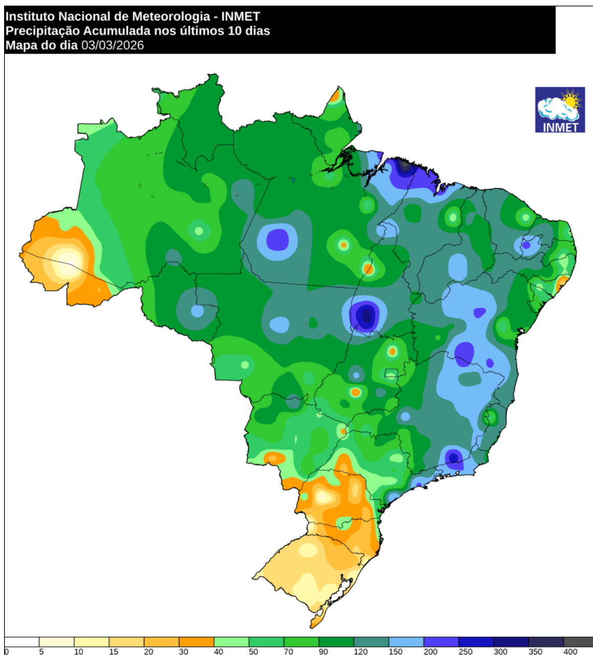
Figura 5a - Pluviometria acumulada (mm) entre os dias 21/02 e 02/03 de 2026. Fonte: INMET.
