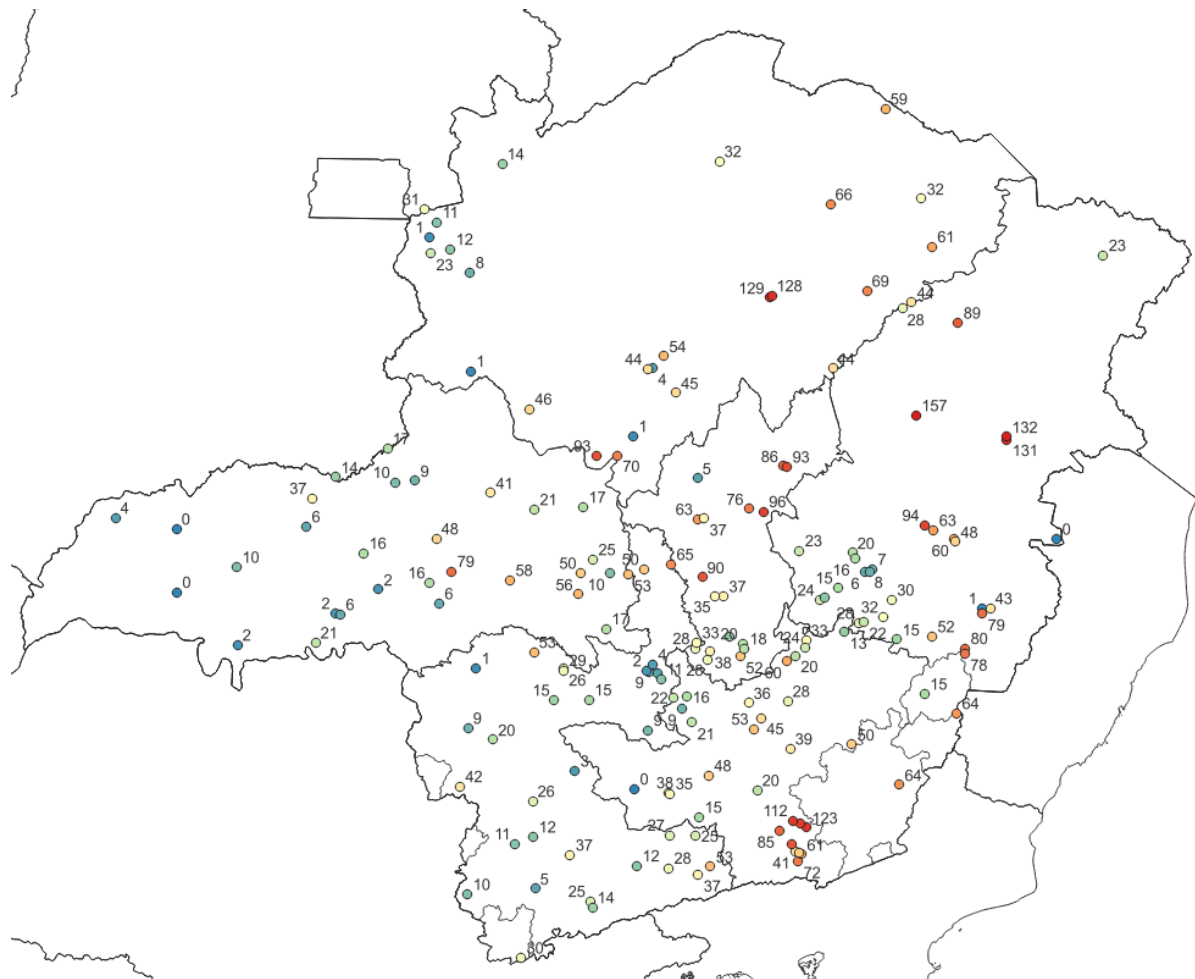
Figura 5b - Pluviometria acumulada entre os dias 26 e 28 de fevereiro de 2026. Fonte dos dados: INMET e CEMIG.
