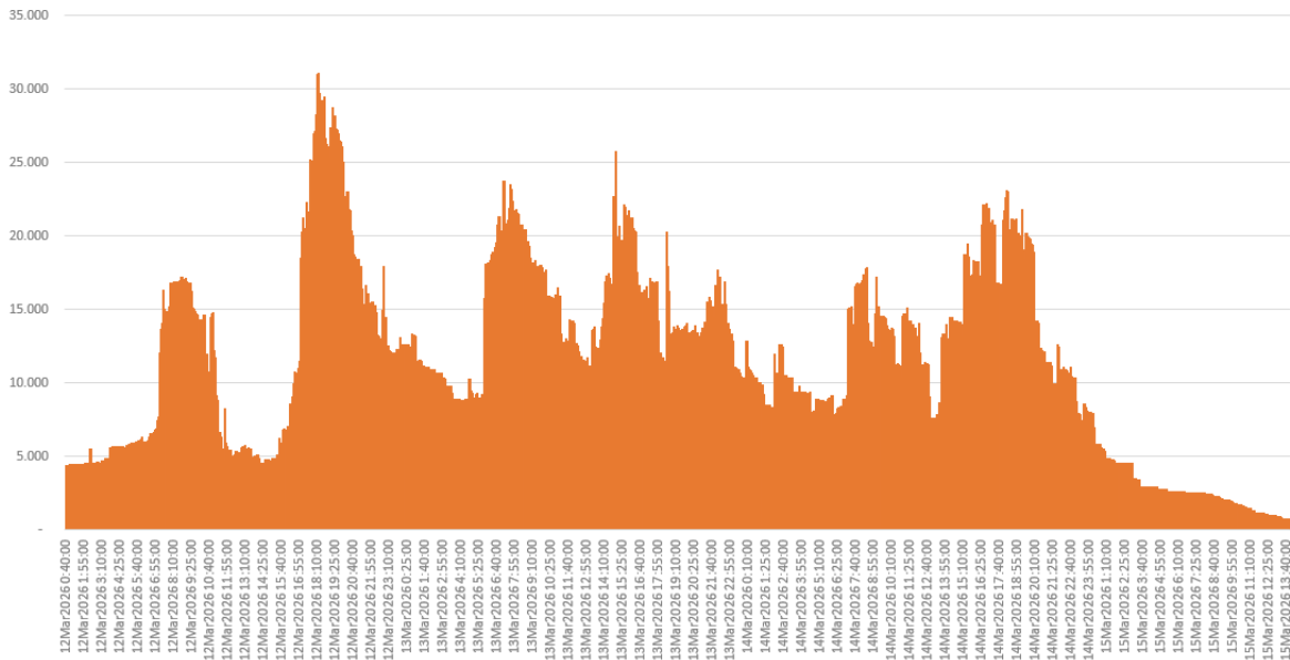
Curva Cliente Interrompido
