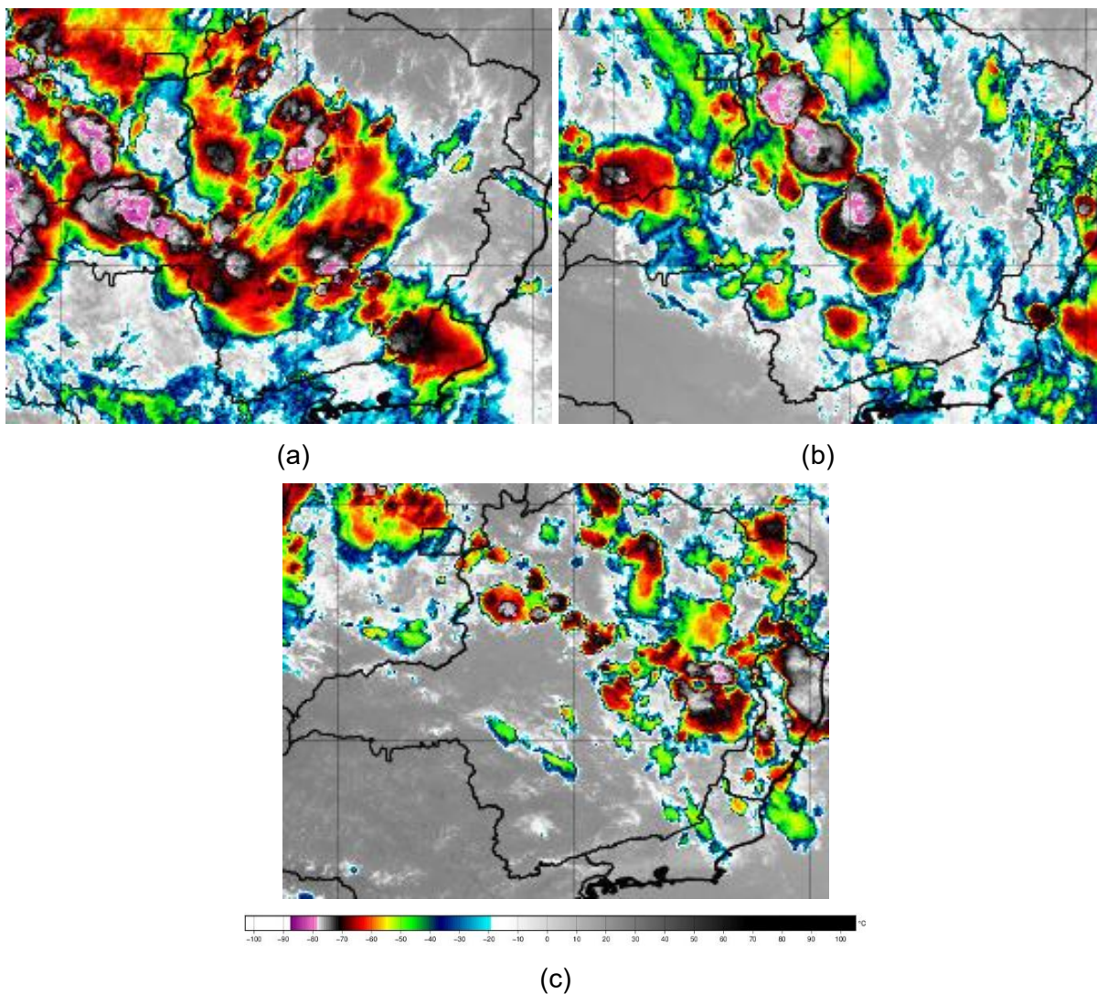
Figura 2 – Seleção de Imagem de Satélite dos dias 12 (a), 13 (b) e 14 (c) de março de 2026. Fonte: INPE.
