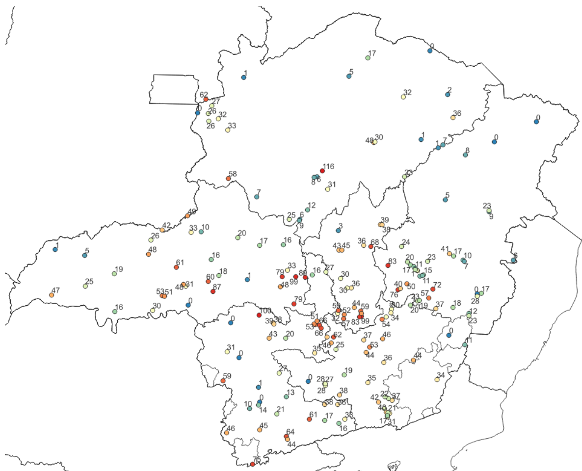
Figura 5b - Pluviometria acumulada entre os dias 12 e 14 de março de 2026. Fonte dos dados: INMET e CEMIG.
