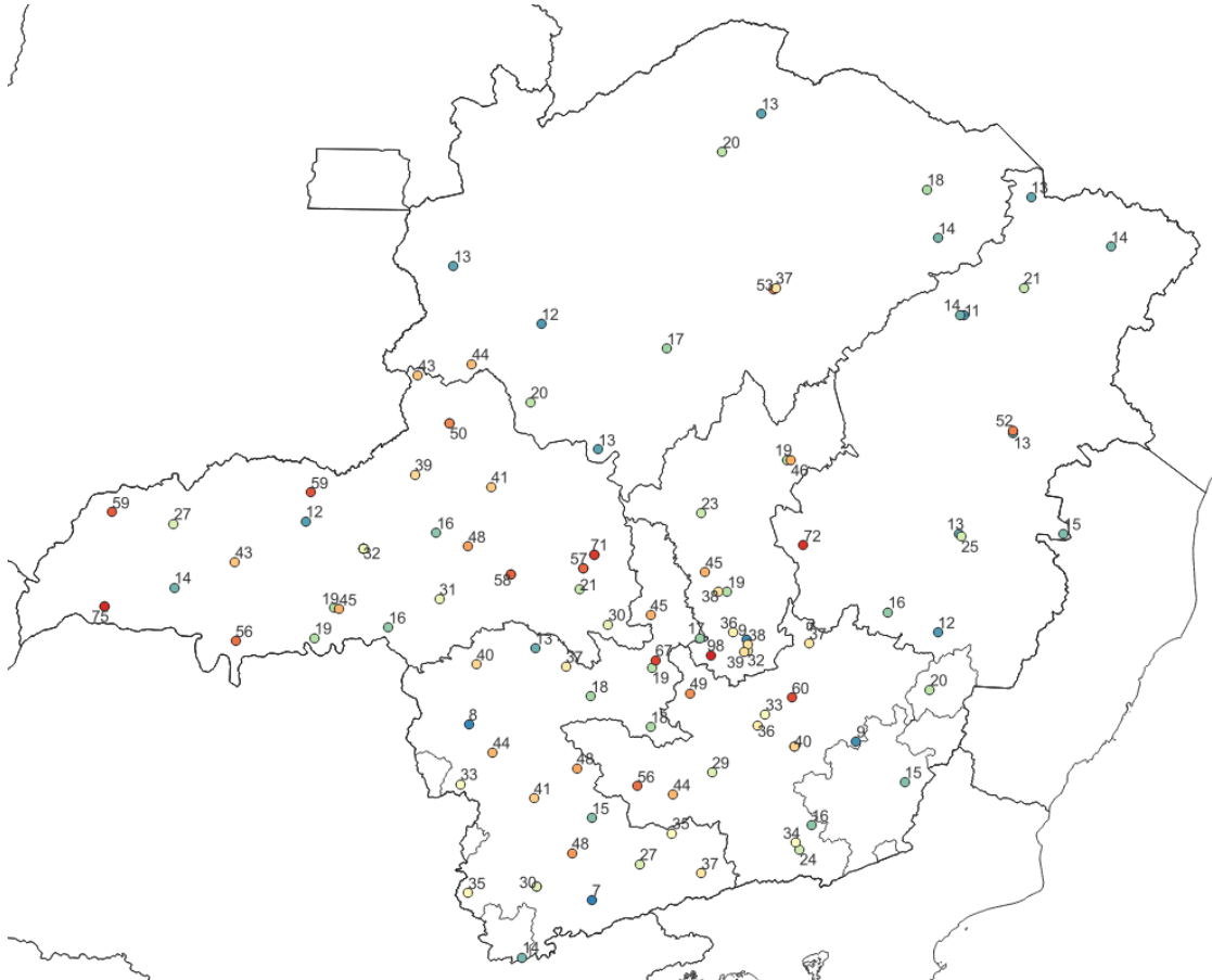
Figura 4 – Rajadas de vento (Km/h) máximas registradas entre os dias 12 e 14 de março de 2026. Fonte: INMET
