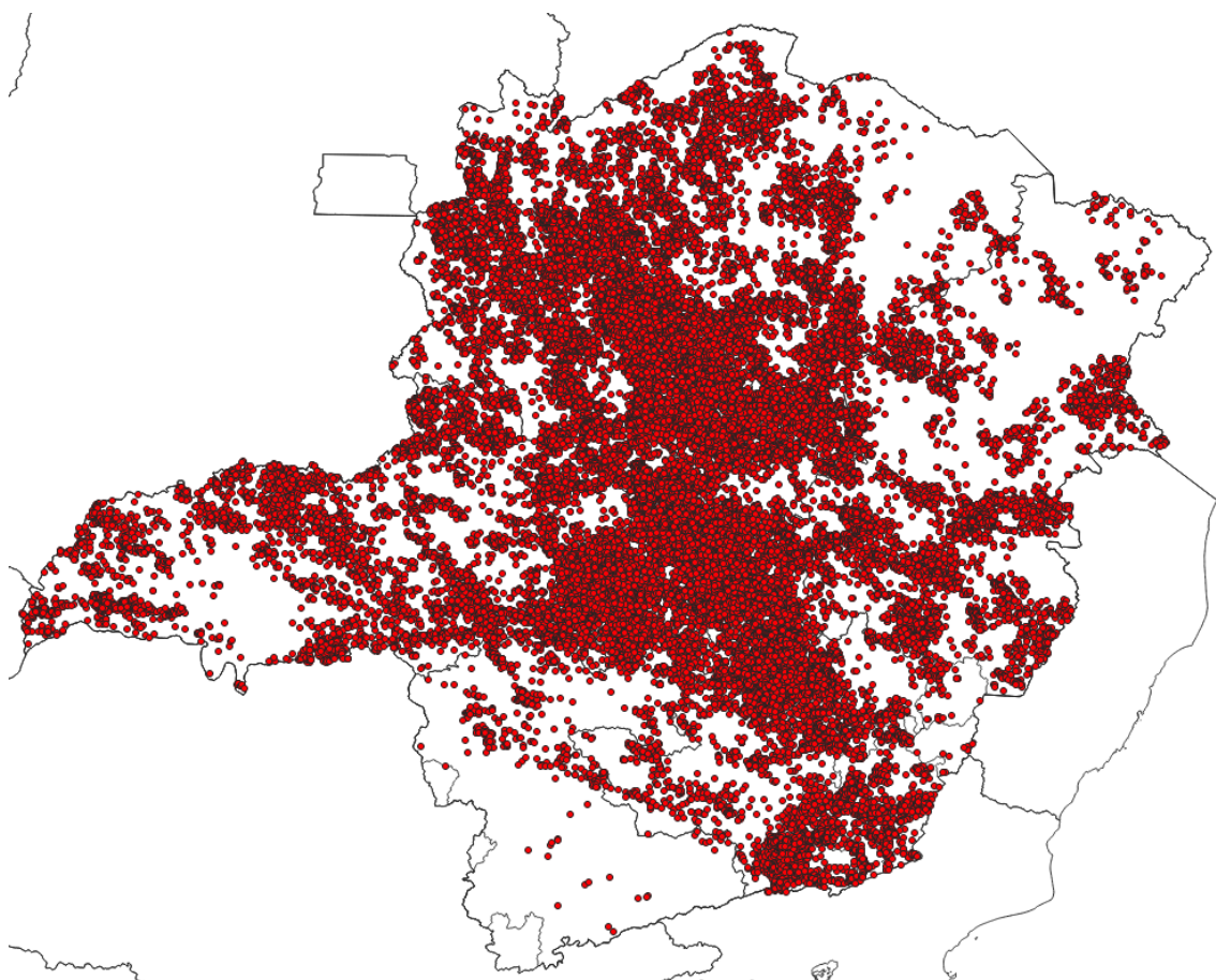
Figura 3 - Localização dos raios registrados entre os dias 12 e 14 de março de 2026. Fonte: RINDAT
