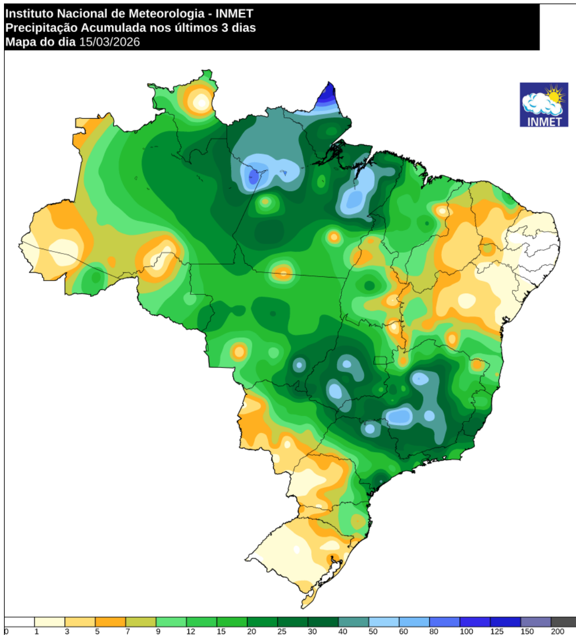
Figura 5a - Pluviometria acumulada (mm) entre os dias 12 e 14 de março de 2026. Fonte: INMET.
