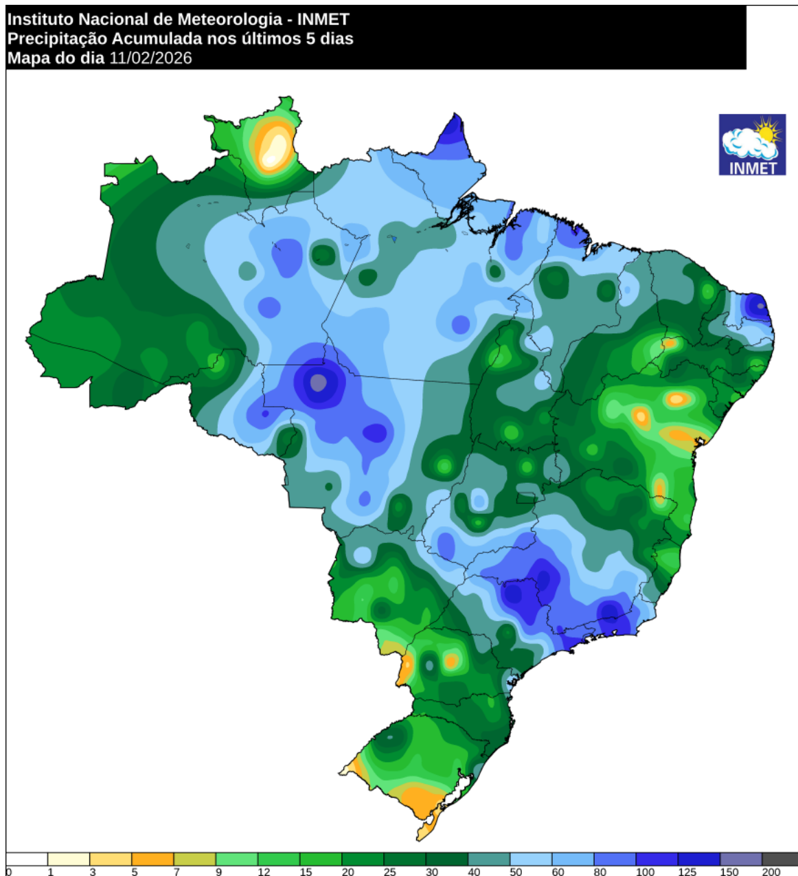
Figura 5a - Pluviometria acumulada (mm) entre os dias 06 e 10 de fevereiro de 2026. Fonte: INMET.
