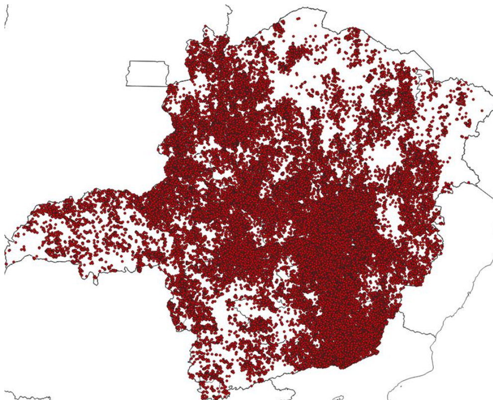
Figura 3 - Localização dos raios registrados entre os dias 07 e 10 de fevereiro de 2026. Fonte: RINDAT
