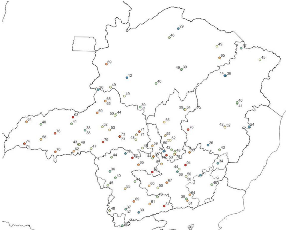
Figura 4 – Rajadas de vento (Km/h) máximas registradas entre os dias 07 e 10 de fevereiro de 2026. Fonte: INMET e CEMIG
