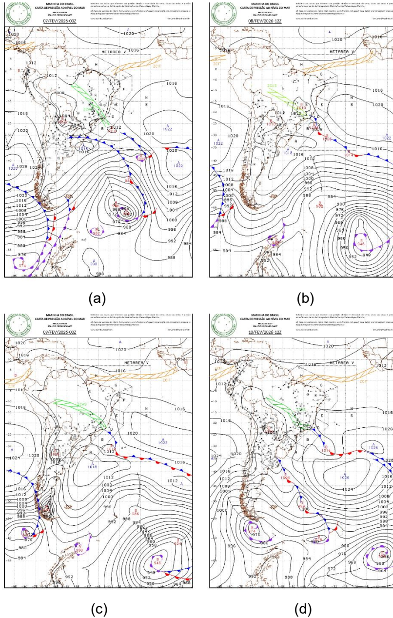
Figura 1 - Carta Sinótica em superfície dos dias 07 (a), 08 (b), 09 (c) e 10 (d) de fevereiro de 2026. Fonte: Marinha do Brasil.
