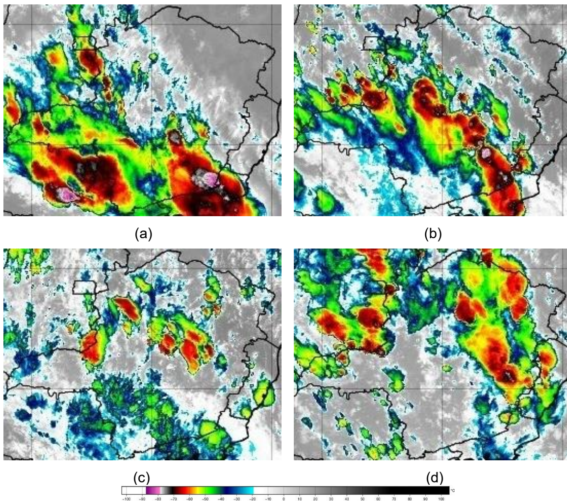
Figura 2 – Seleção de Imagens de Satélite dos dias 07 (a), 08 (b), 09 (c) e 10 (d) de fevereiro de 2026. Fonte: INPE.
