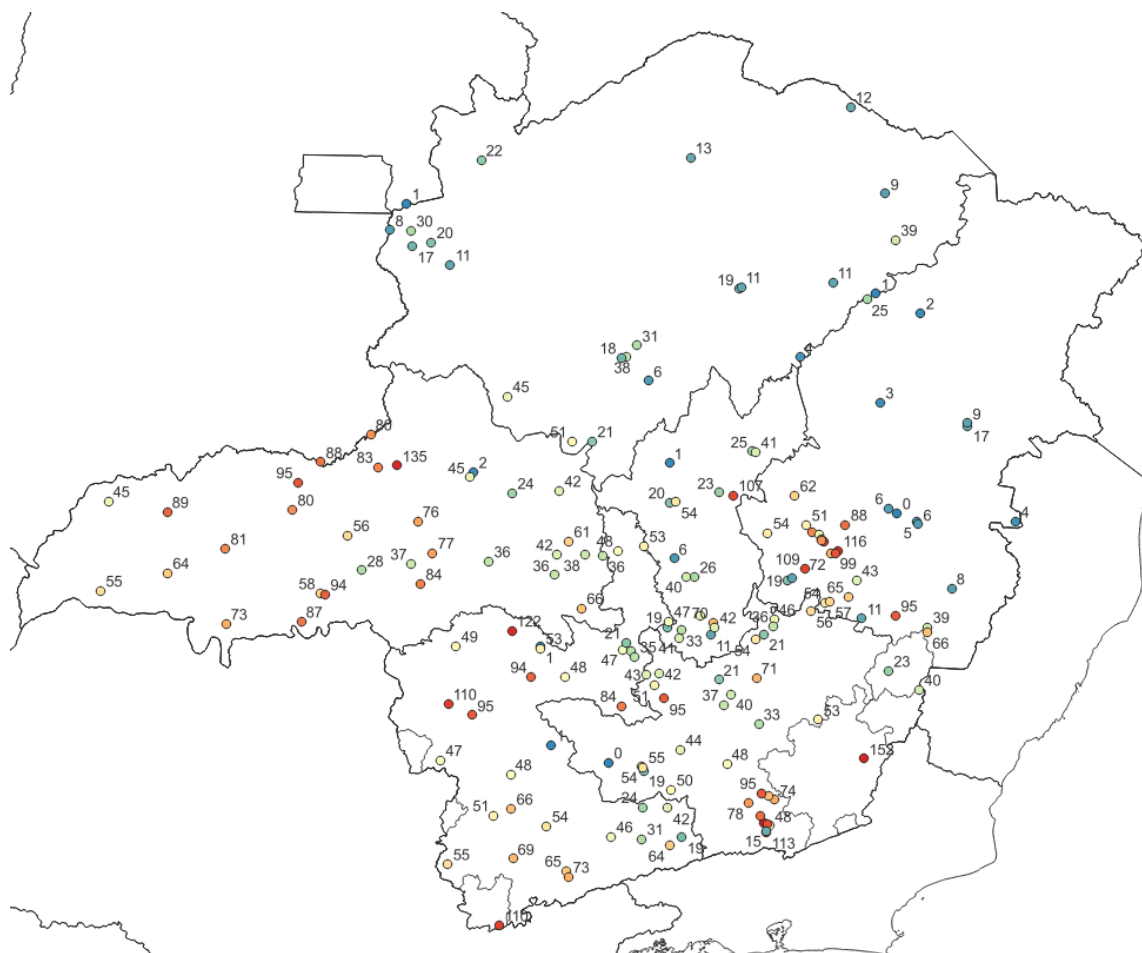
Figura 5b - Pluviometria acumulada entre os dias 07 e 10 de fevereiro de 2026. Fonte dos dados: INMET e CEMIG.
