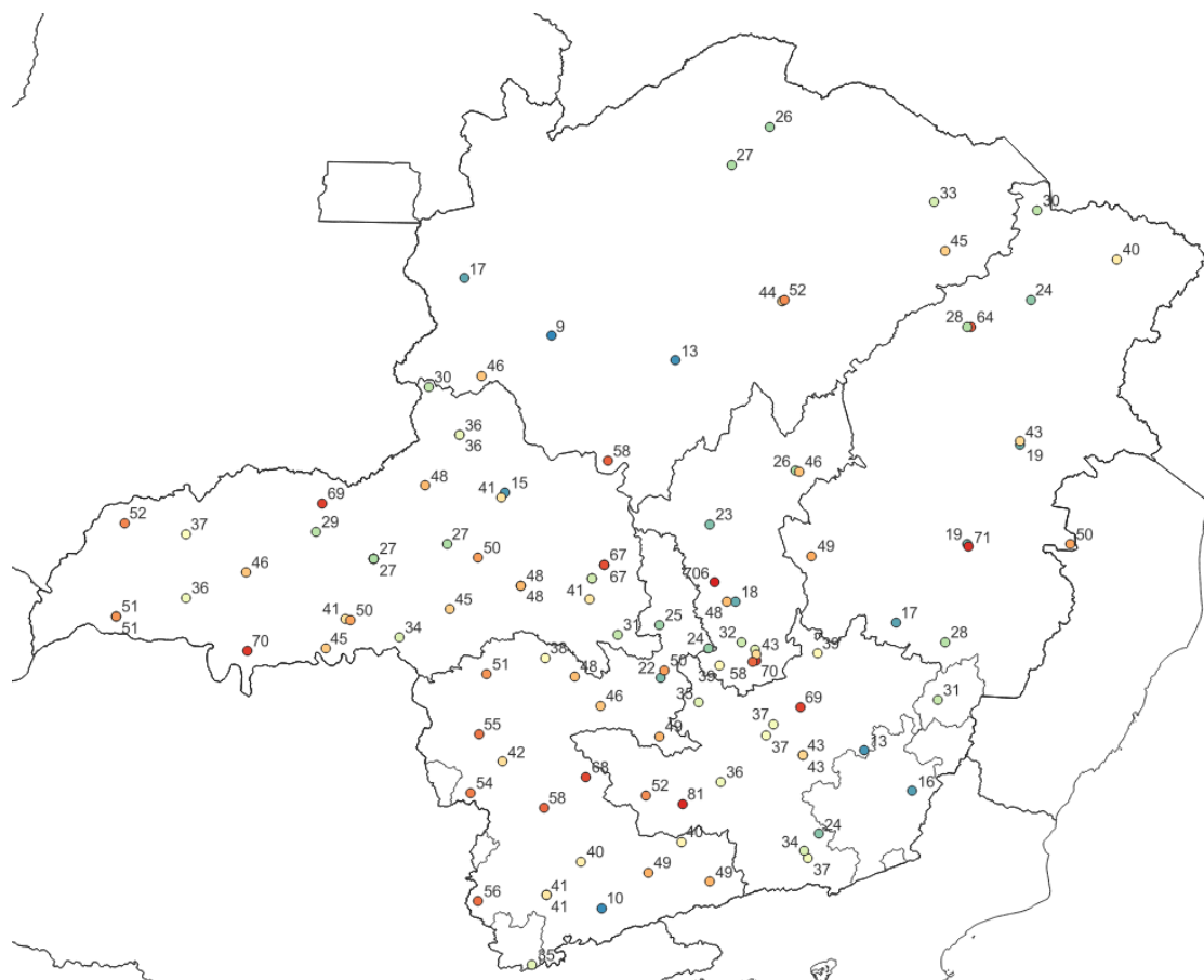
Figura 4 – Rajadas de vento (Km/h) máximas registradas entre os dias 03 e 06 de janeiro de 2026. Fonte: INMET e CEMIG
