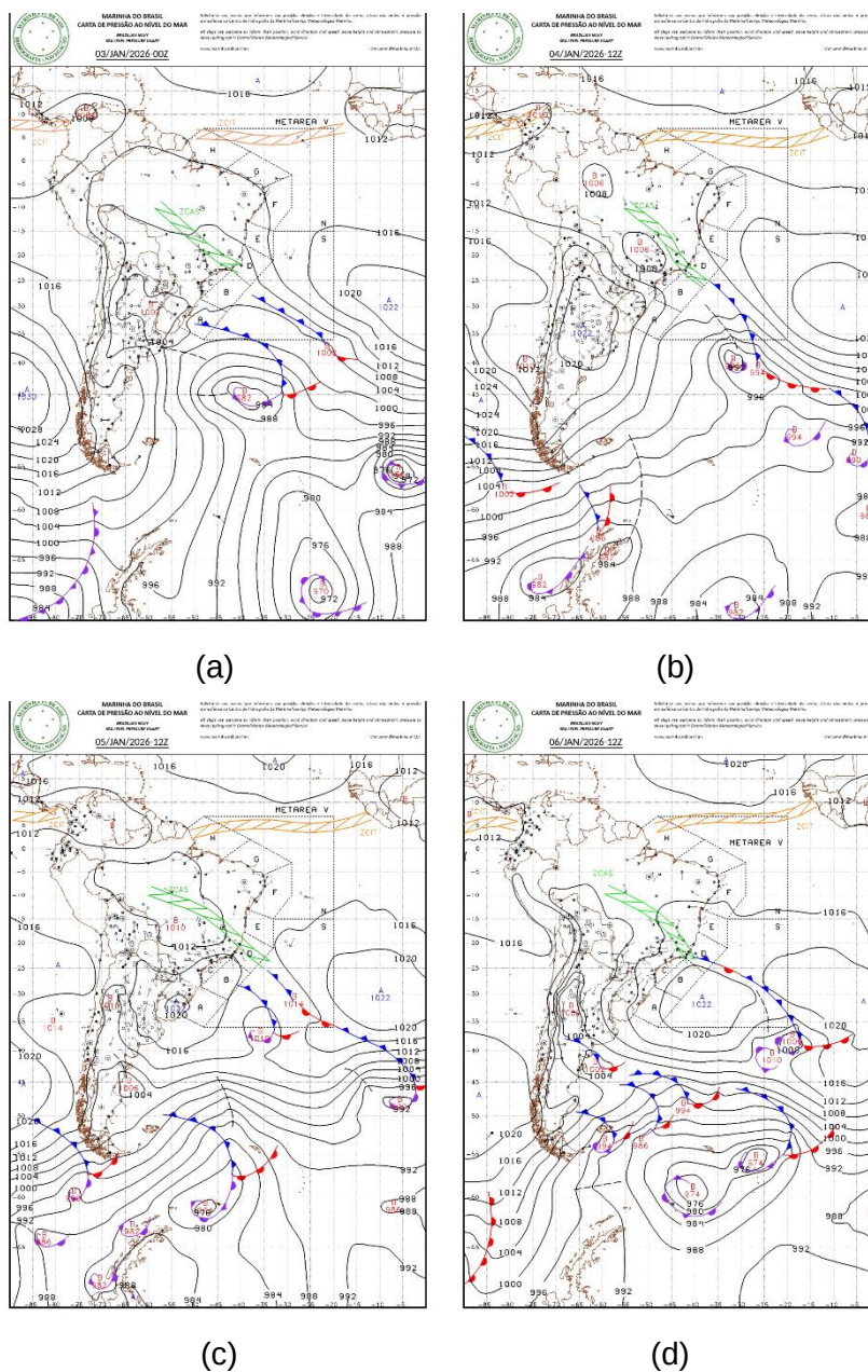
Figura 1 - Carta Sinótica em superfície dos dias 03 (a), 04 (b), 05 (c) e 06 (d) de janeiro de 2026. Fonte: Marinha do Brasil.
