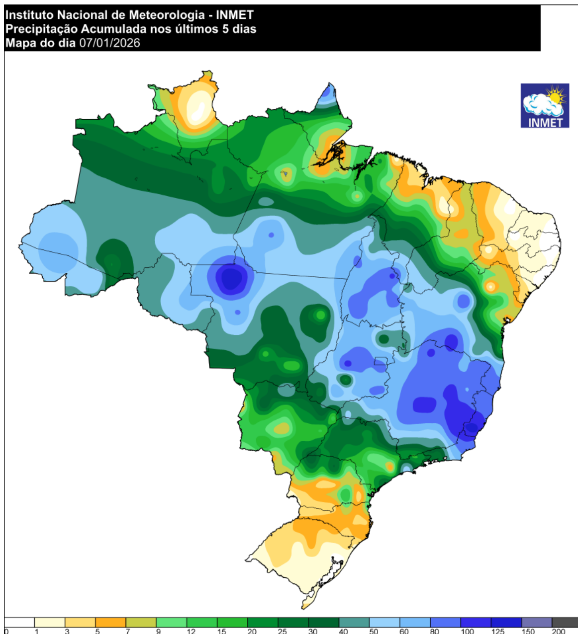
Figura 5a - Pluviometria acumulada (mm) entre os dias 02 e 06 de janeiro de 2026. Fonte: INMET.
