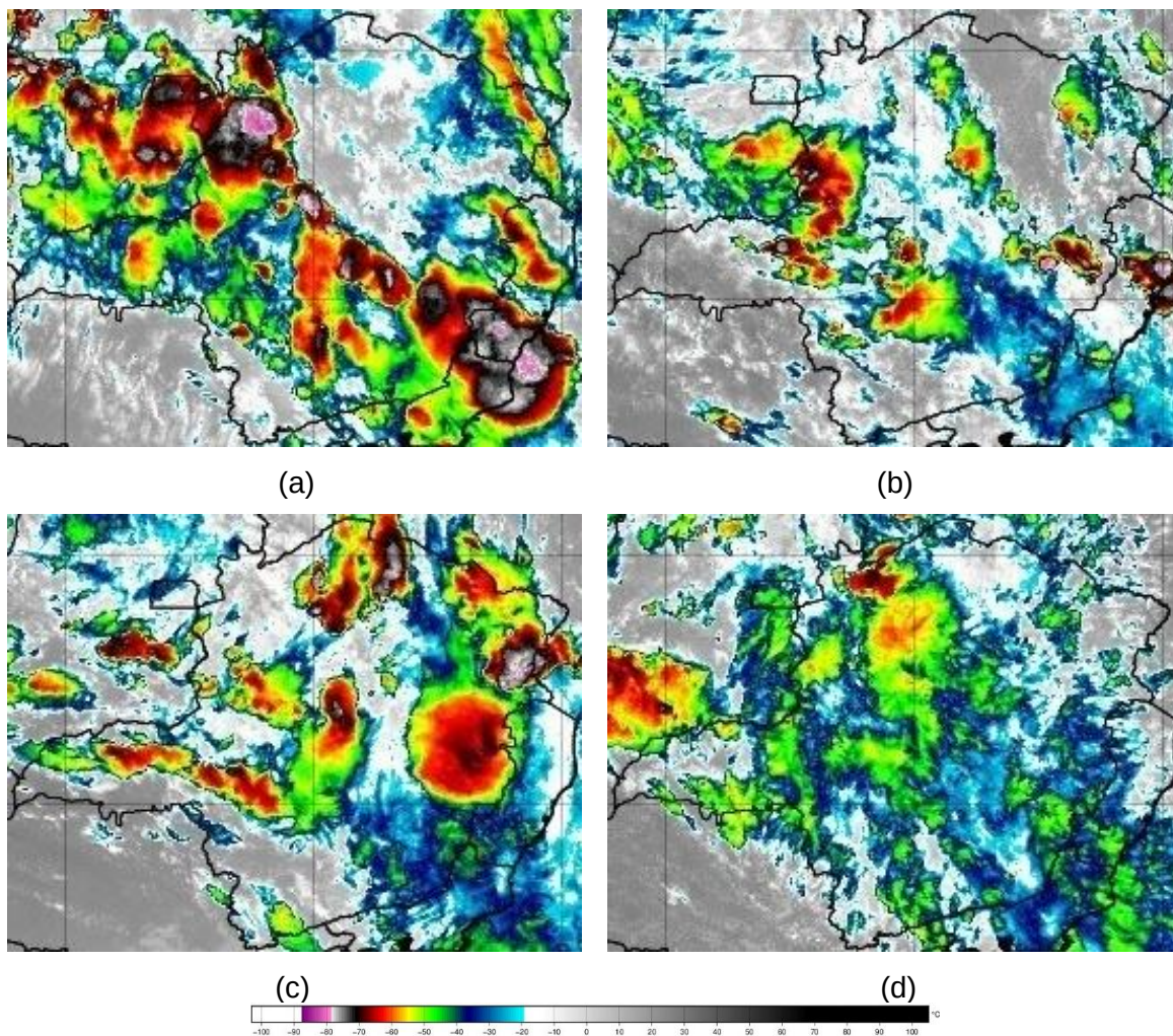
Figura 2 – Seleção de Imagens de Satélite dos dias 03 (a), 04 (b), 05 (c) e 06 (d) de janeiro de 2026. Fonte: INPE.
