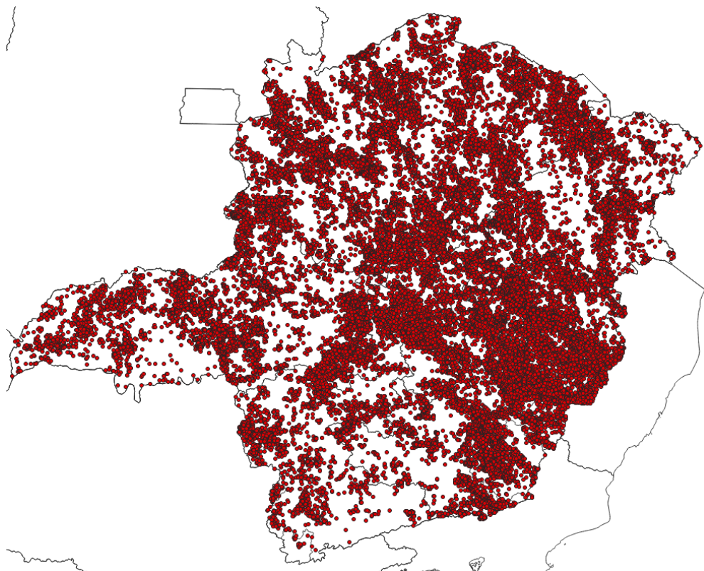
Figura 3 - Localização dos raios registrados entre os dias 03 e 06 de janeiro de 2026. Fonte: RINDAT
