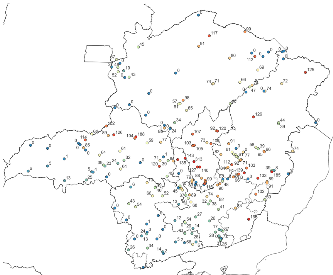
Figura 5b - Pluviometria acumulada entre os dias 03 e 06 de janeiro de 2026. Fonte dos dados: INMET e CEMIG.
