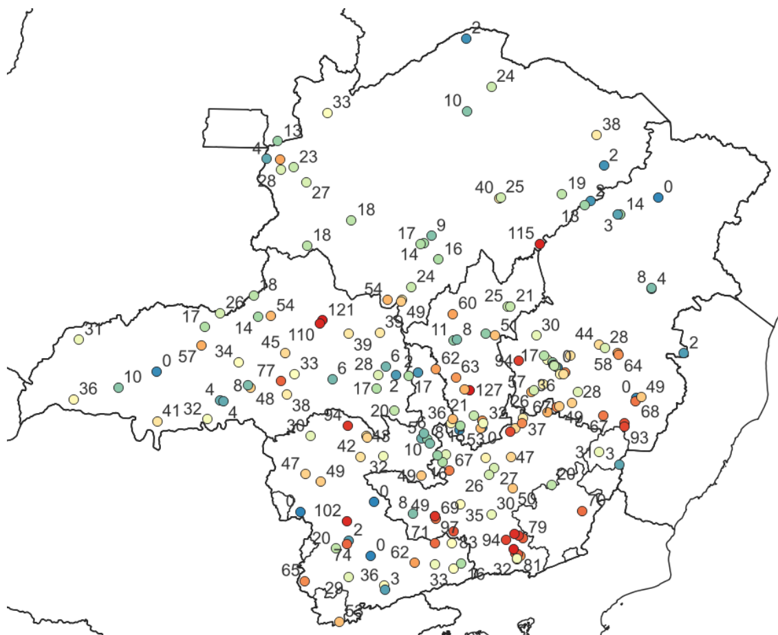
Figura 5b - Pluviometria acumulada entre os dias 12 e 15 de dezembro de 2025. Fonte dos dados: INMET e CEMIG.
