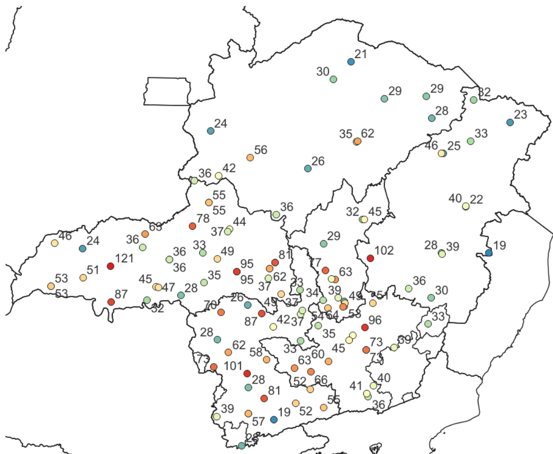
Figura 4 – Rajadas de vento (Km/h) máximas registradas entre os dias 12 e 15 de dezembro de 2025. Fonte: INMET e CEMIG
