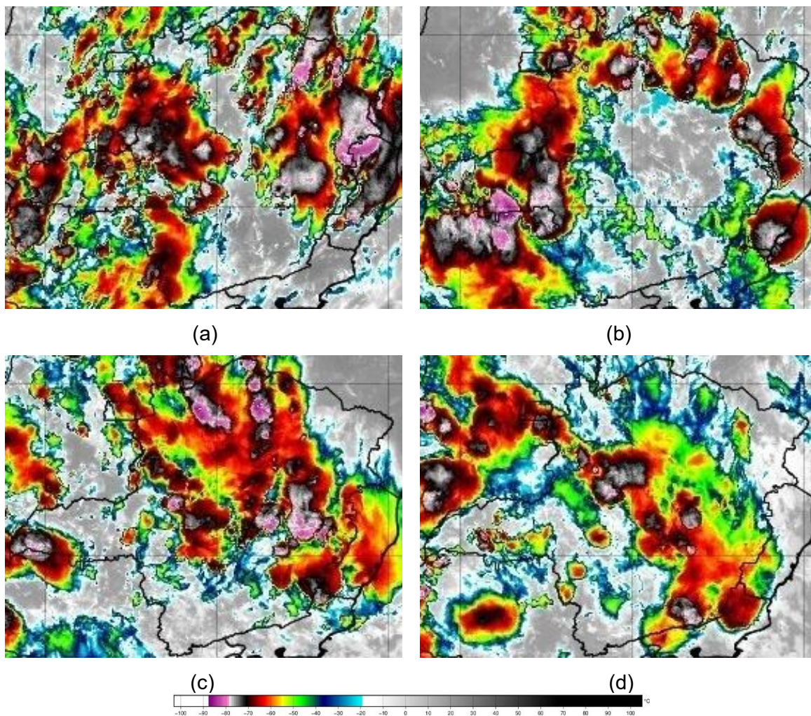
Figura 2 – Seleção de Imagens de Satélite dos dias 12 (a), 13 (b), 14 (c) e 15 (d) de dezembro de 2025. Fonte: INPE.
