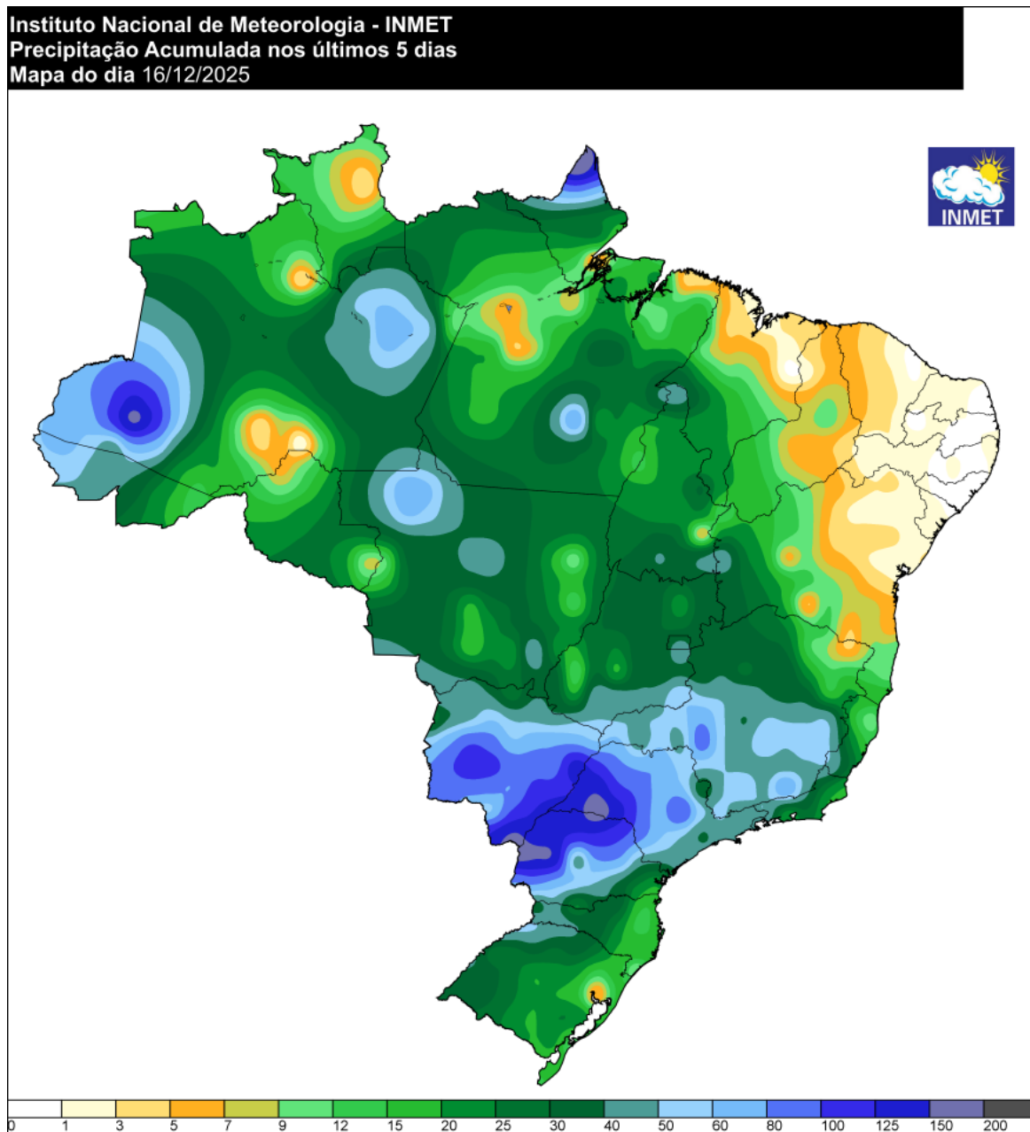
Figura 5a - Pluviometria acumulada (mm) entre os dias 11 e 15 de dezembro de 2025. Fonte: INMET.
