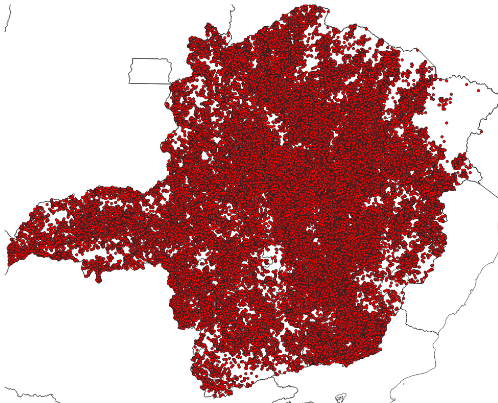
Figura 3 - Localização dos raios registrados entre os dias 12 e 15 de dezembro de 2025. Fonte: RINDAT
