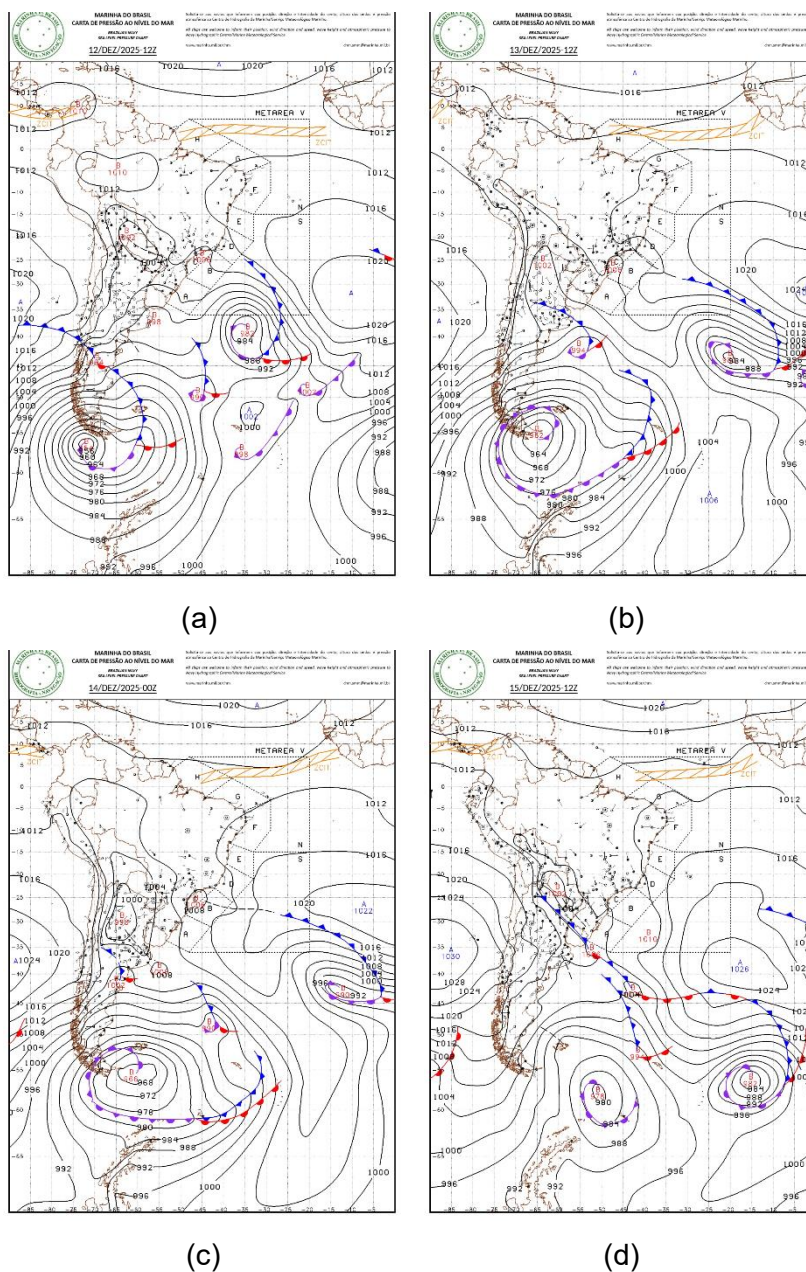
Figura 1 - Carta Sinótica em superfície dos dias 12 (a), 13 (b), 14 (c) e 15 (d) de dezembro de 2025. Fonte: Marinha do Brasil.
