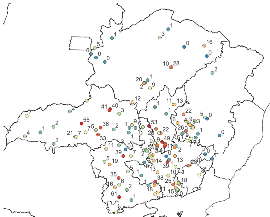
Figura 5b - Pluviometria acumulada entre os dias 01 e 02 de dezembro de 2025. Fonte dos dados: INMET e CEMIG.
