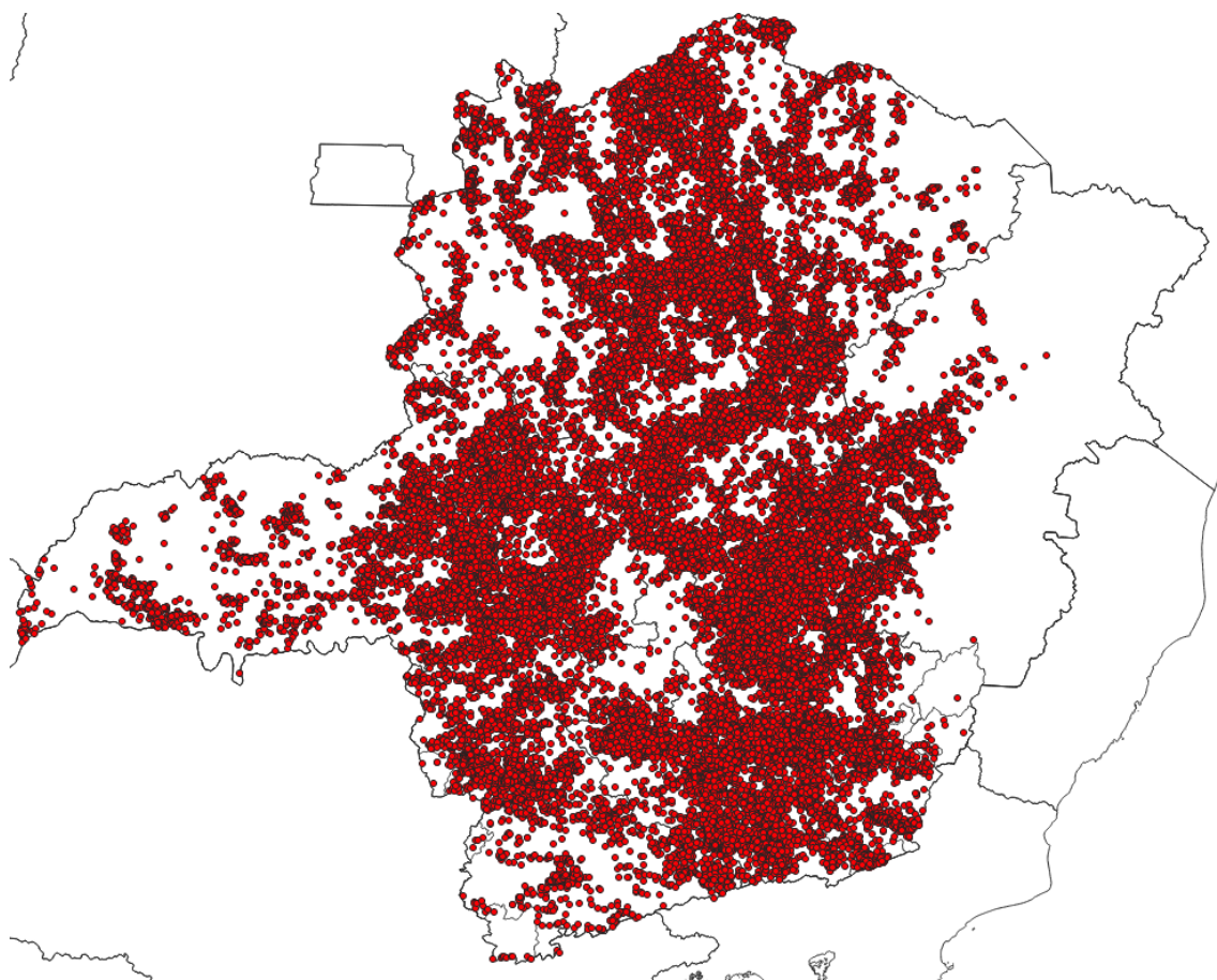
Figura 3 - Localização dos raios registrados entre os dias 01 e 02 de dezembro de 2025. Fonte: RINDAT
