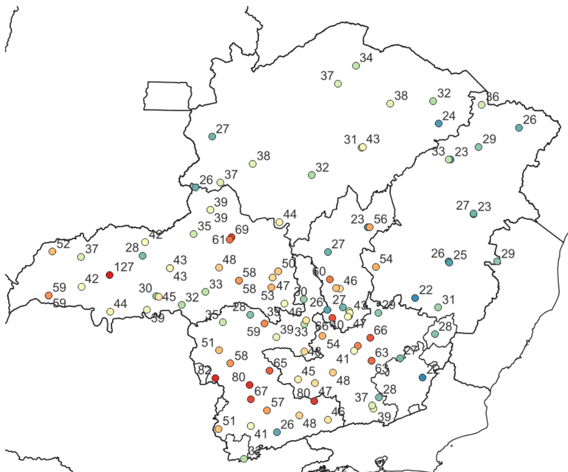
Figura 4 – Rajadas de vento (Km/h) máximas registradas entre os dias 01 e 02 de dezembro de 2025. Fonte: INMET e CEMIG
