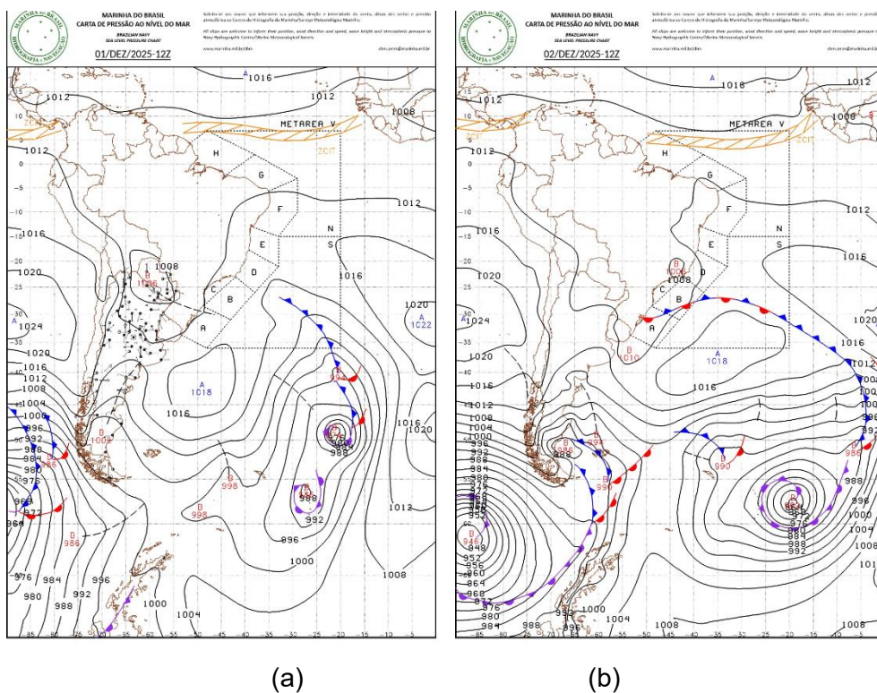
Figura 1 - Carta Sinótica em superfície dos dias 01 (a) e 02 (b) de dezembro de 2025. Fonte: Marinha do Brasil.
