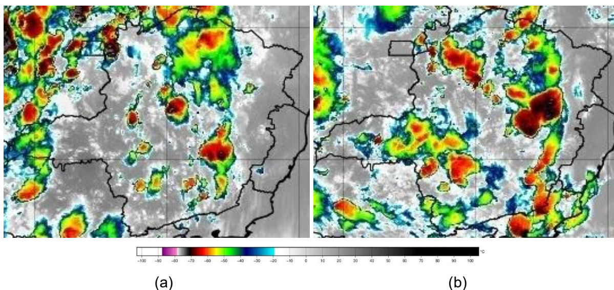
Figura 2 – Seleção de Imagem de Satélite dos dias 01 (a) e 02 (b) de dezembro de 2025. Fonte: INPE.
