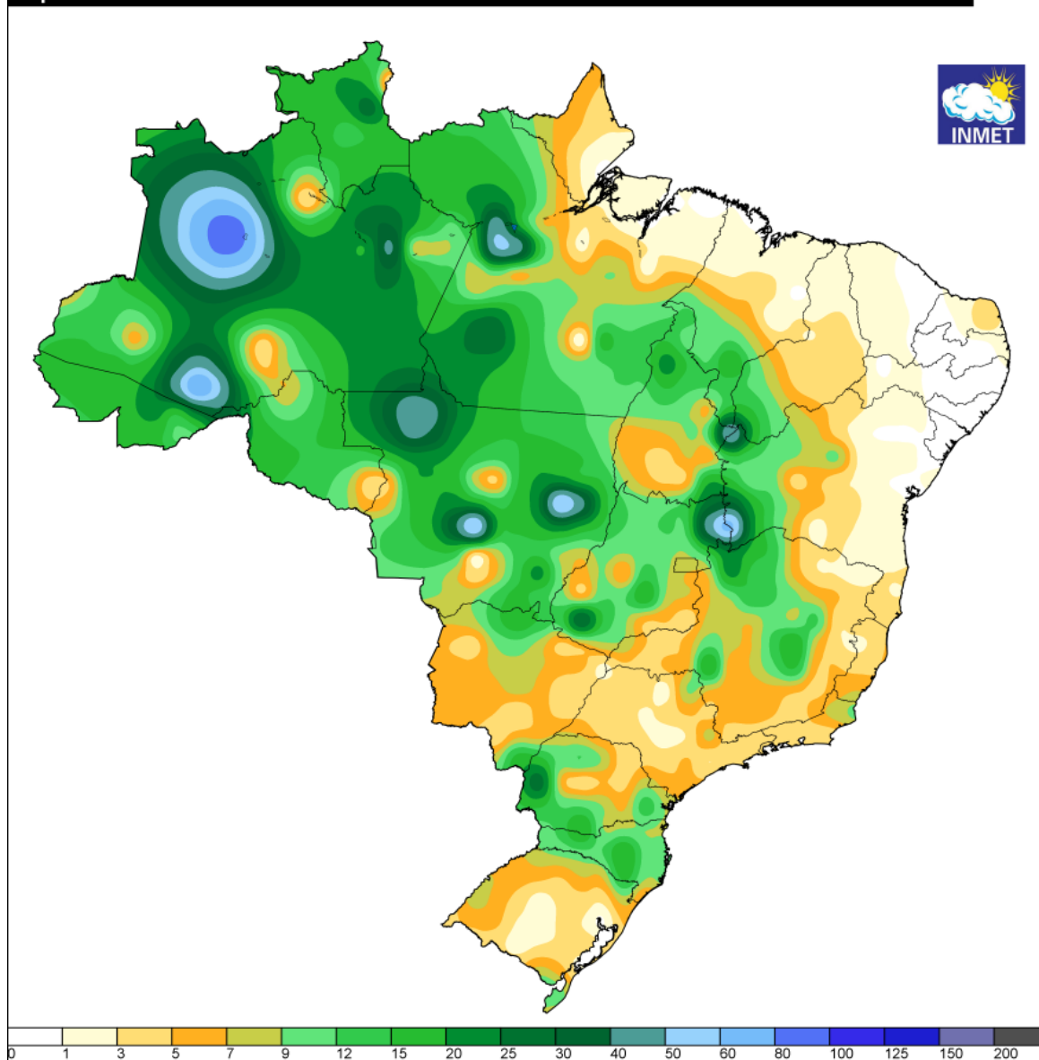
Figura 5a - Pluviometria acumulada (mm) entre os dias 30/11 e 02/12 de 2025. Fonte: INMET.
