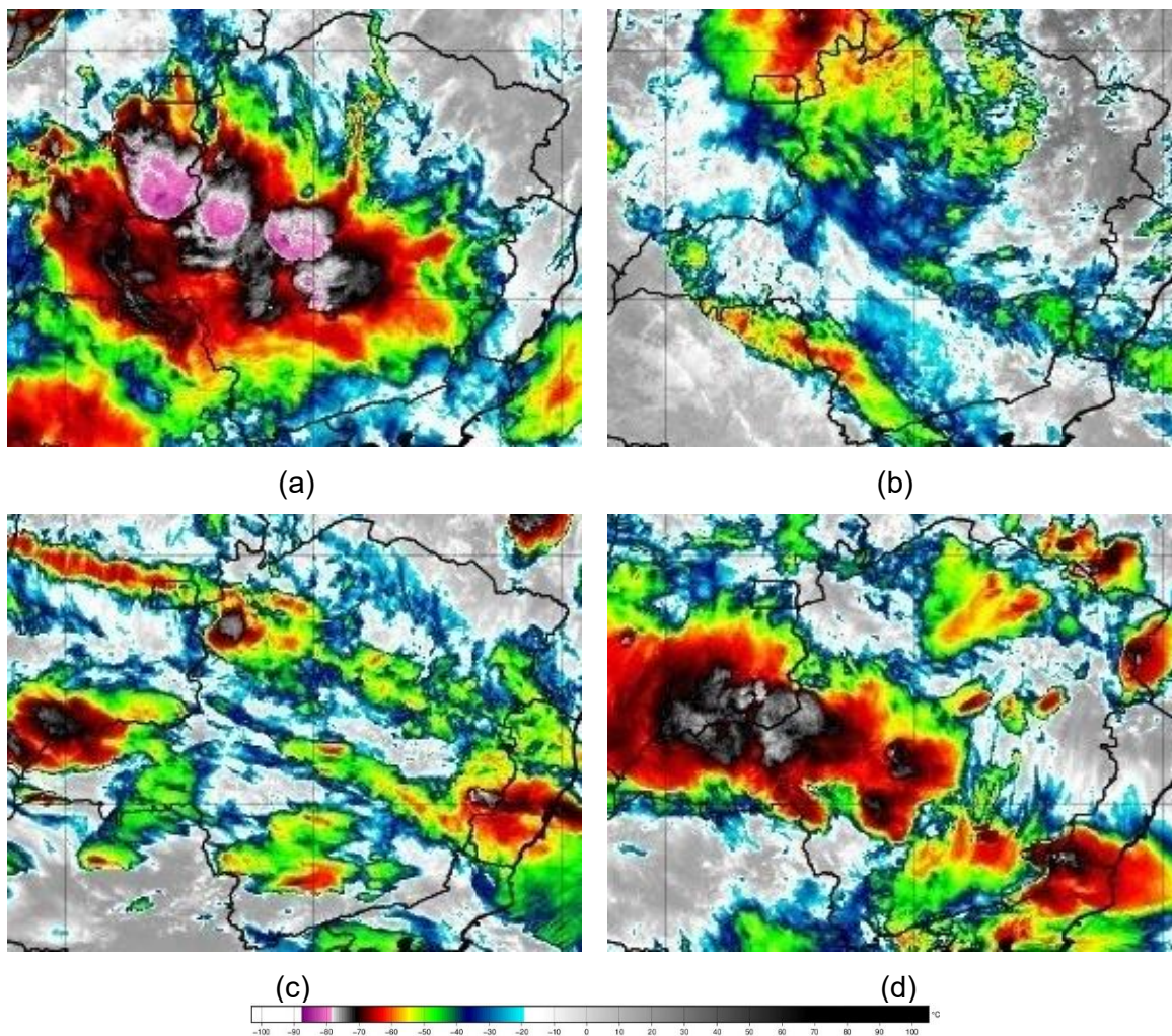
Figura 2 – Seleção de Imagens de Satélite dos dias 02 (a), 03 (b), 04 (c) e 05 (d) de novembro de 2025. Fonte: INPE.
