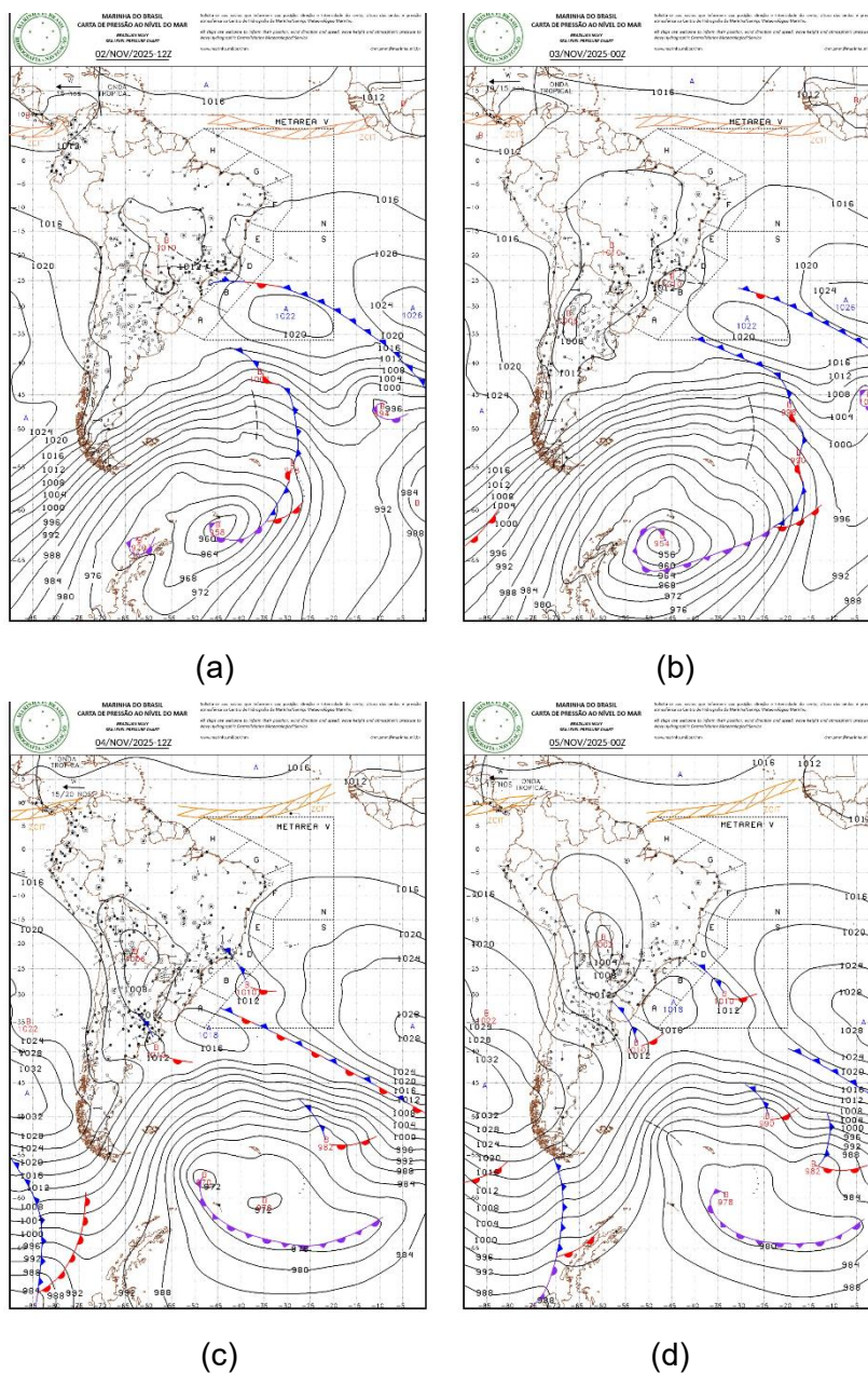
Figura 1 - Carta Sinótica em superfície dos dias 02 (a), 03 (b), 04 (c) e 05 (d) de novembro de 2025. Fonte: Marinha do Brasil.
