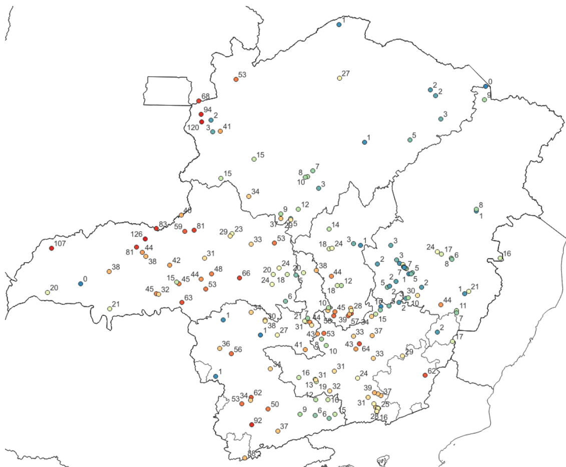
Figura 5b - Pluviometria acumulada entre os dias 02 e 05 de novembro de 2025 . Fonte dos dados: INMET e CEMIG.
