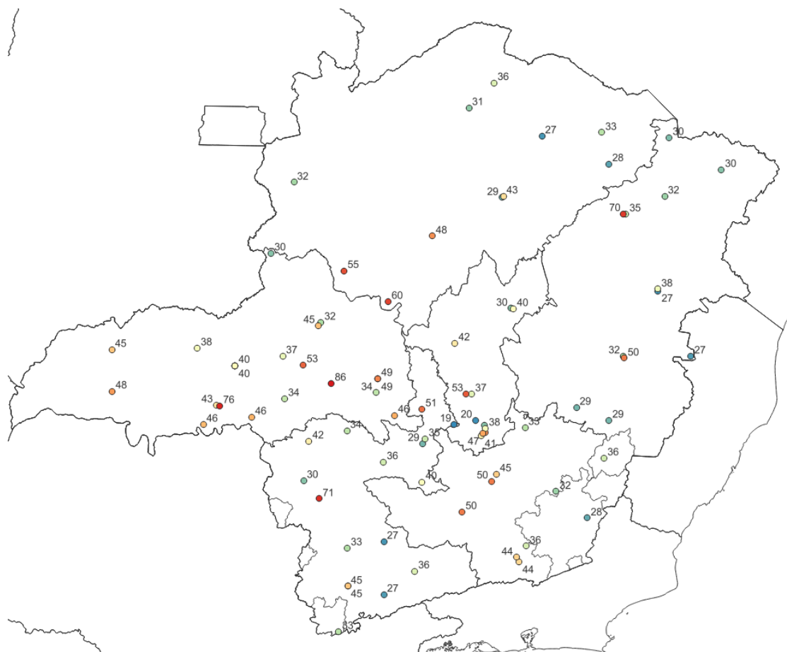
Figura 4 – Rajadas de vento (Km/h) máximas registradas entre os dias 02 e 05 de novembro de 2025 . Fonte: INMET e CEMIG
