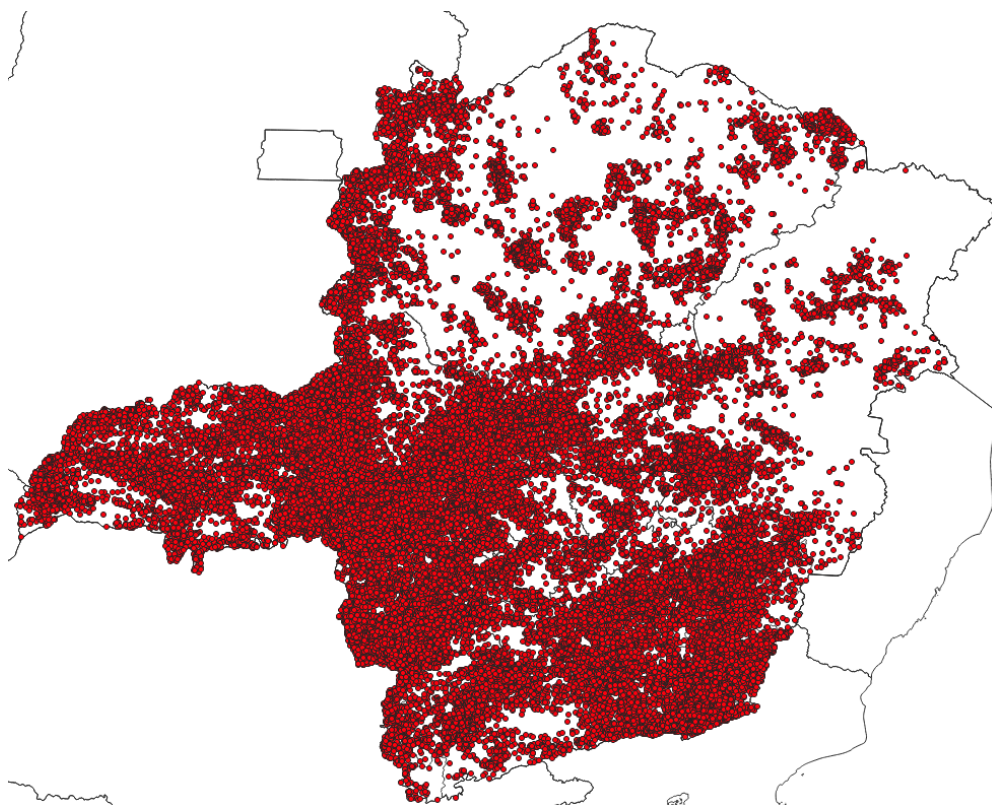
Figura 3 - Localização dos raios registrados entre os dias 02 e 05 de novembro de 2025. Fonte: RINDAT
