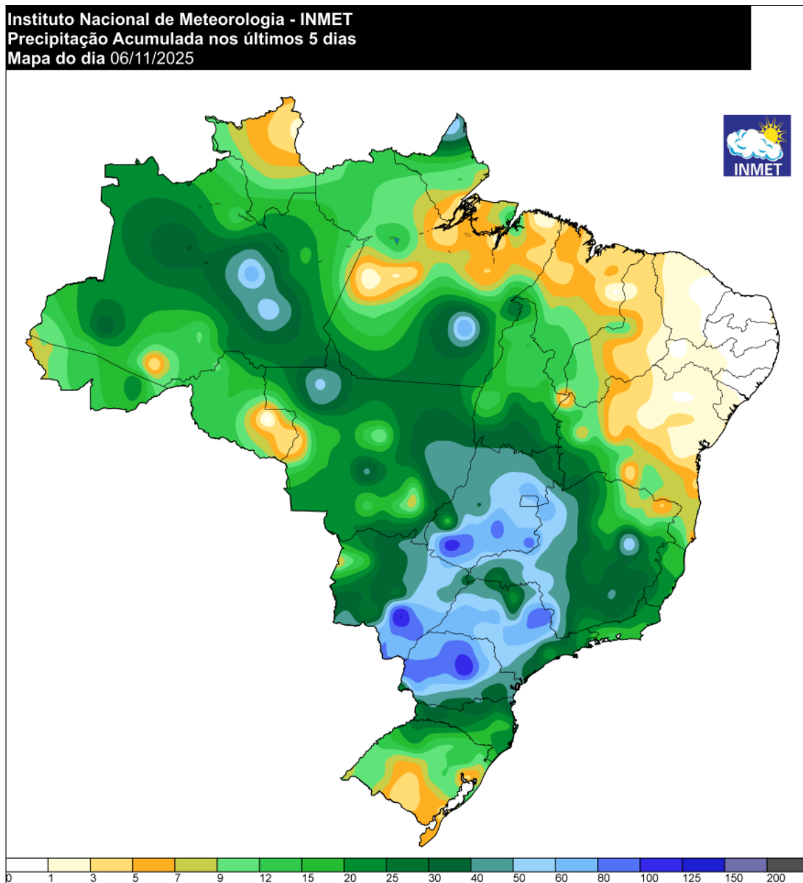
Figura 5a - Pluviometria acumulada (mm) entre os dias 01 e 05 de novembro de 2025. Fonte: INMET.
