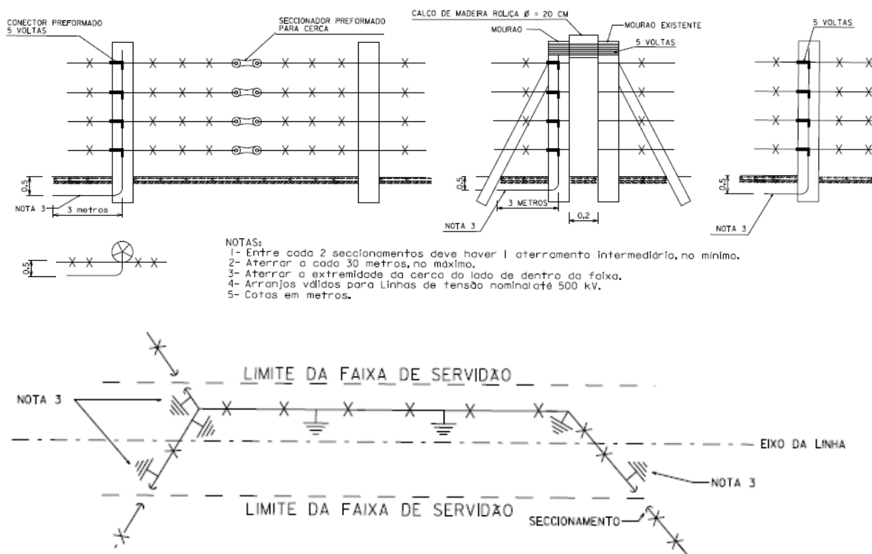
Figura 12. Aterramento e seccionamento de partes metálicas (30.000-ER/LT-2687)
