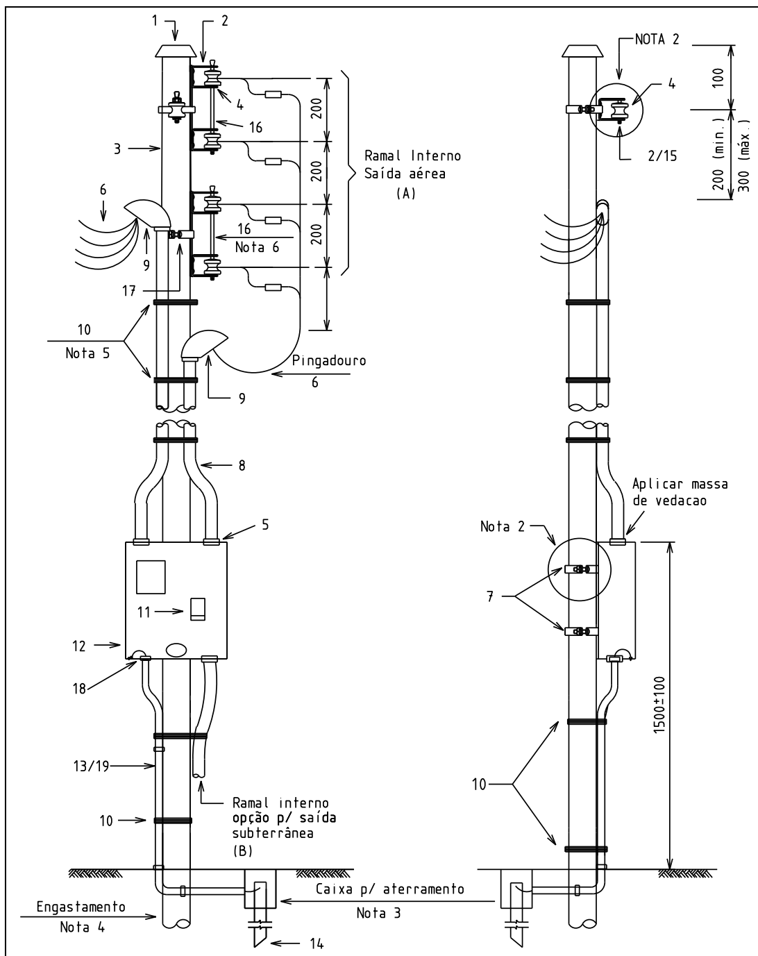
DESENHO 13 - PADRÃO COM RAMAL DE CONEXÃO AÉREO - LIGAÇÃO A 2, 3 e 4 FIOS - INSTALAÇÃO EM POSTE – LEITURA PELA VIA PÚBLICA - CAIXA TIPO CM-1, CM-2, CM-3 OU CM-19
