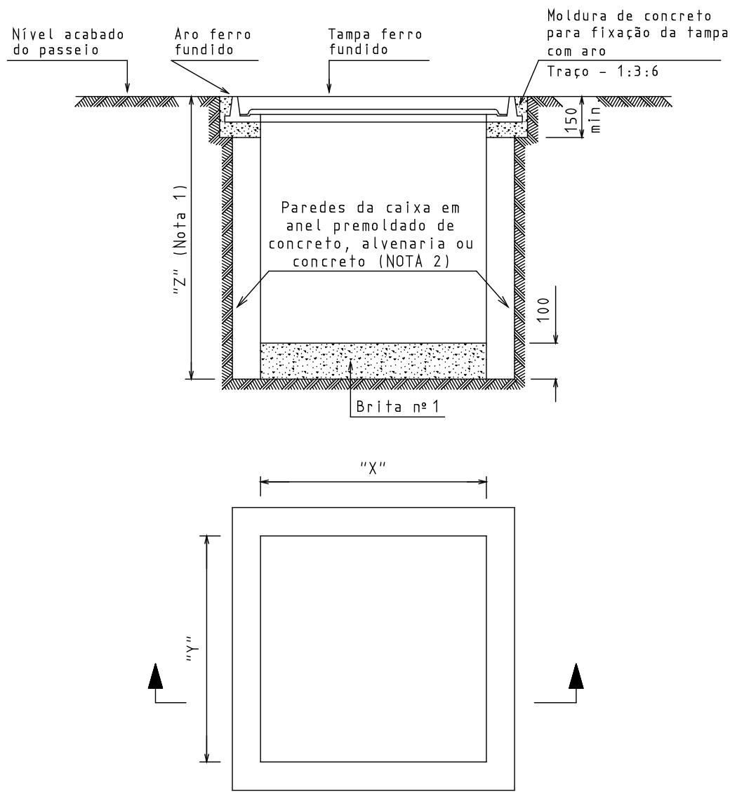
DESENHO 47 - MODELO DE CAIXA DE INSPEÇÃO
