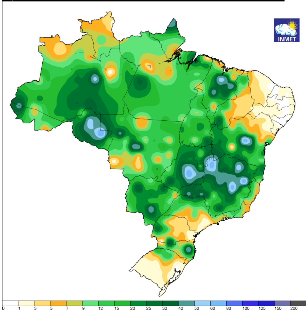
Figura 5a - Pluviometria acumulada (mm) entre os dias 06 e 08 de fevereiro de 2024. Fonte: INMET.
