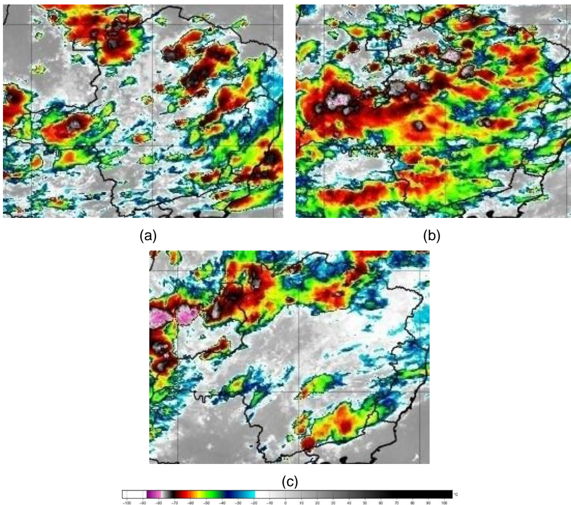
Figura 2 – Seleção de Imagem de Satélite dos dias 06 (a), 07 (b) e 08 (c) de fevereiro de 2024. Fonte: INPE.
