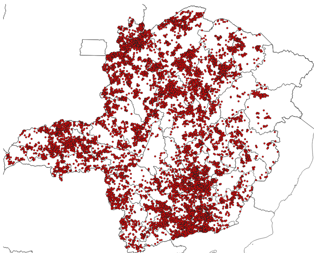
Figura 3 - Localização dos raios registrados entre os dias 06 e 08 de fevereiro de 2024. Fonte: RINDAT
