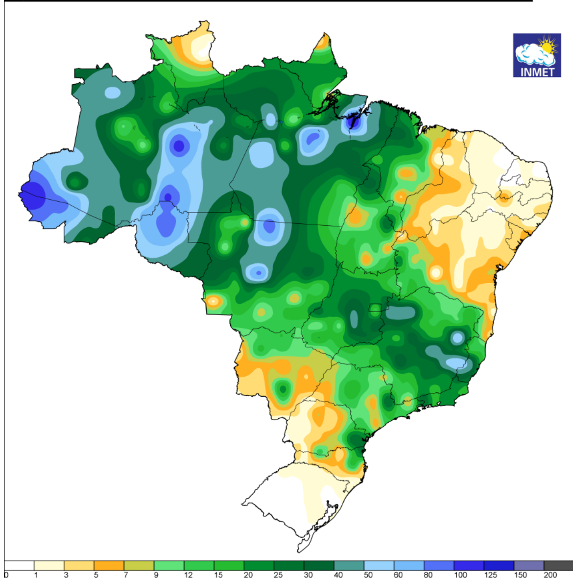
Figura 5a - Pluviometria acumulada (mm) entre os dias 30/01 e 01/02 de 2024. Fonte: INMET.
