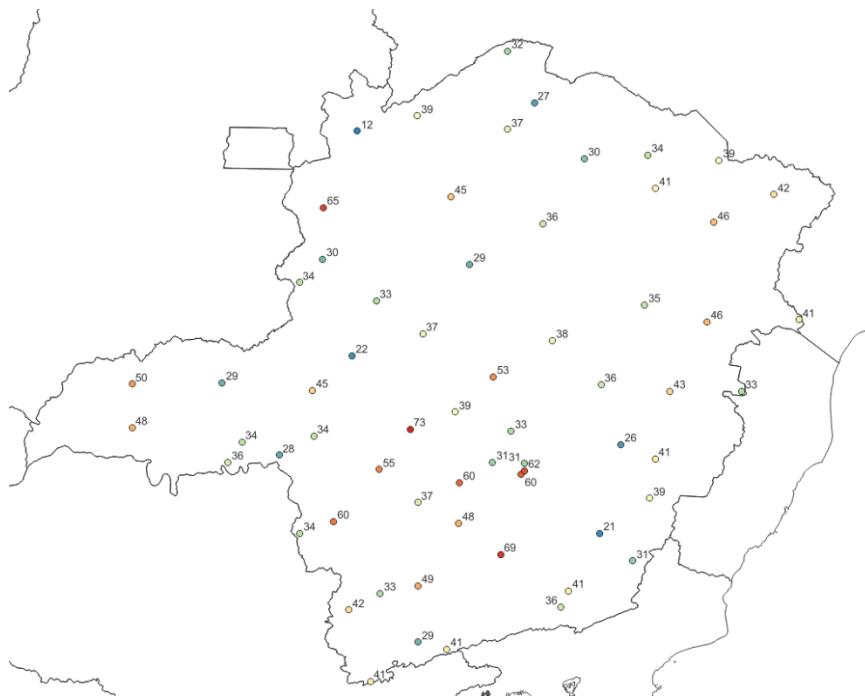
Figura 4 – Rajadas de vento (Km/h) máximas registradas entre os dias 30/01 e 01/02 de 2024. Fonte: INMET
