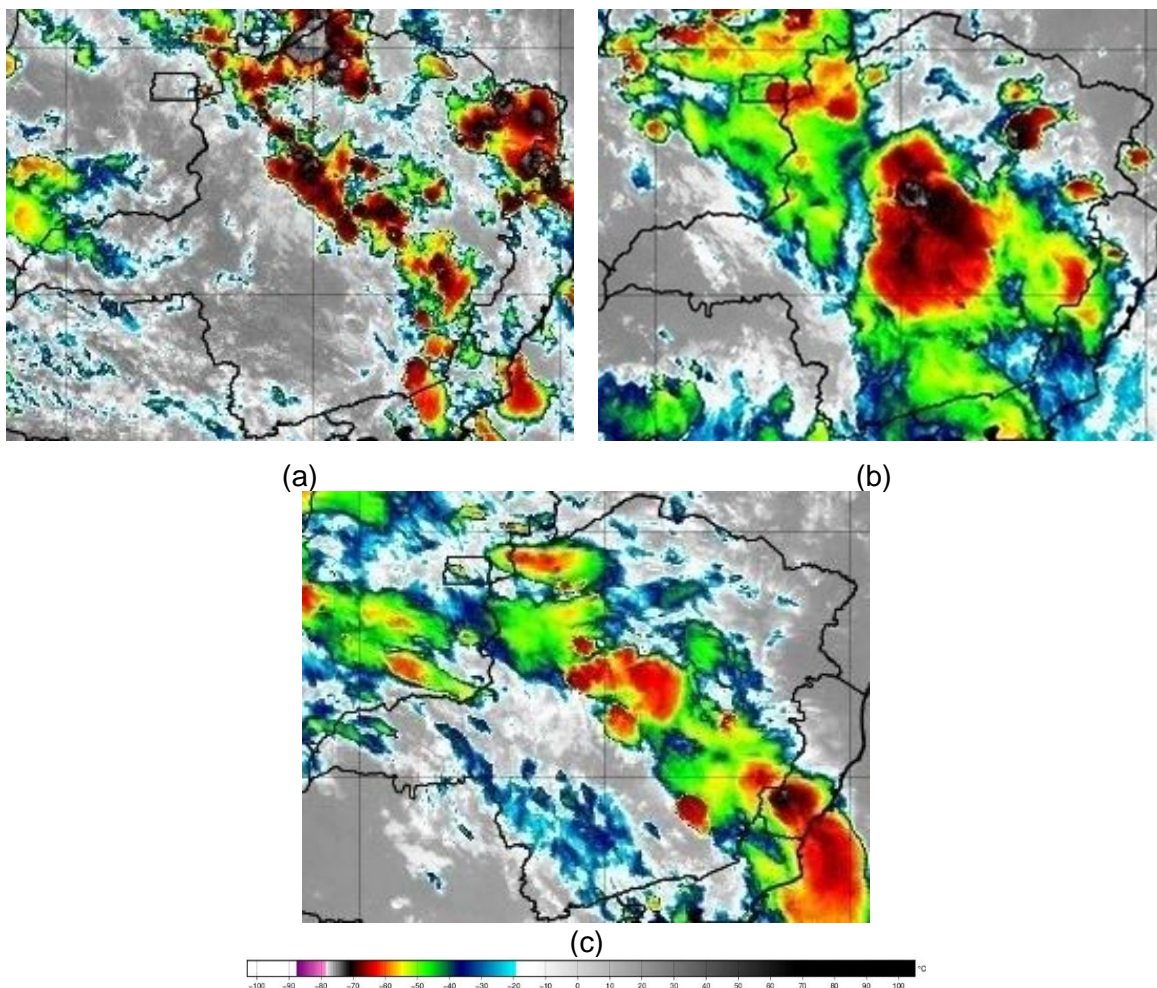
Figura 2 – Seleção de Imagem de Satélite dos dias 30/01 (a) e 01/02 de 2024. Fonte: INPE.
