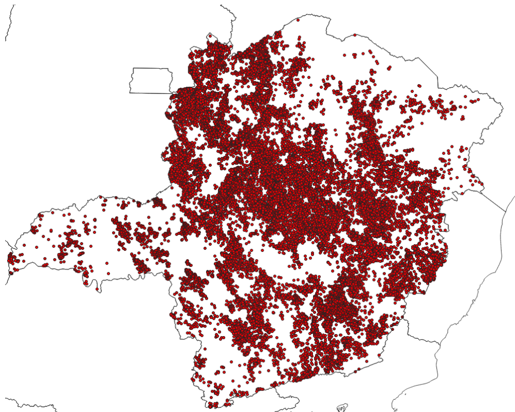
Figura 3 - Localização dos raios registrados entre os dias 30/01 e 01/02 de 2024. Fonte: RINDAT
