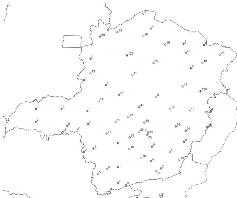
Figura 5b - Pluviometria acumulada entre os dias 30/01 e 01/02 de 2024. Fonte dos dados: INMET.
