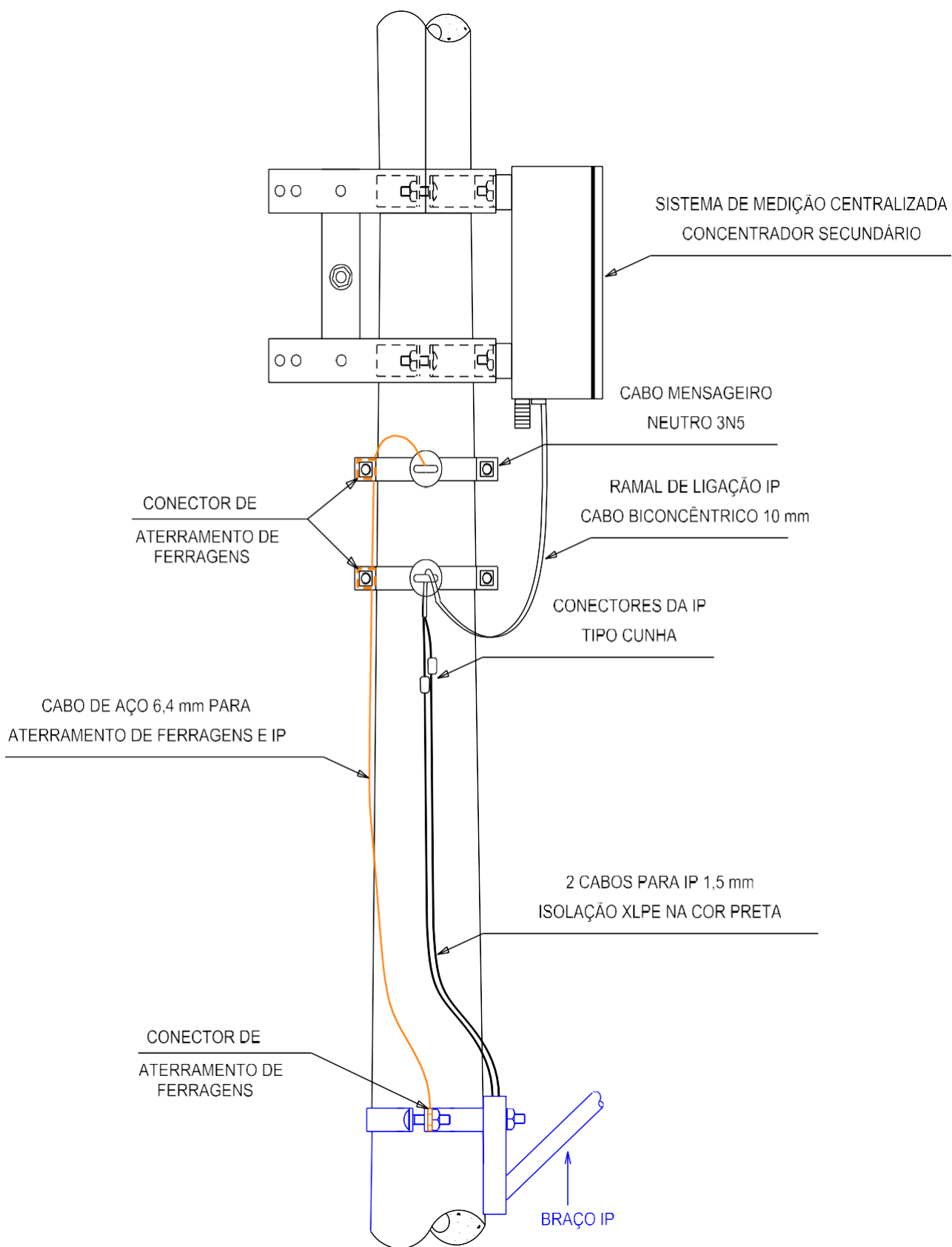
Figura 4 - Aterramento Definitivo de Ferragens e Ligação de Equipamentos de
