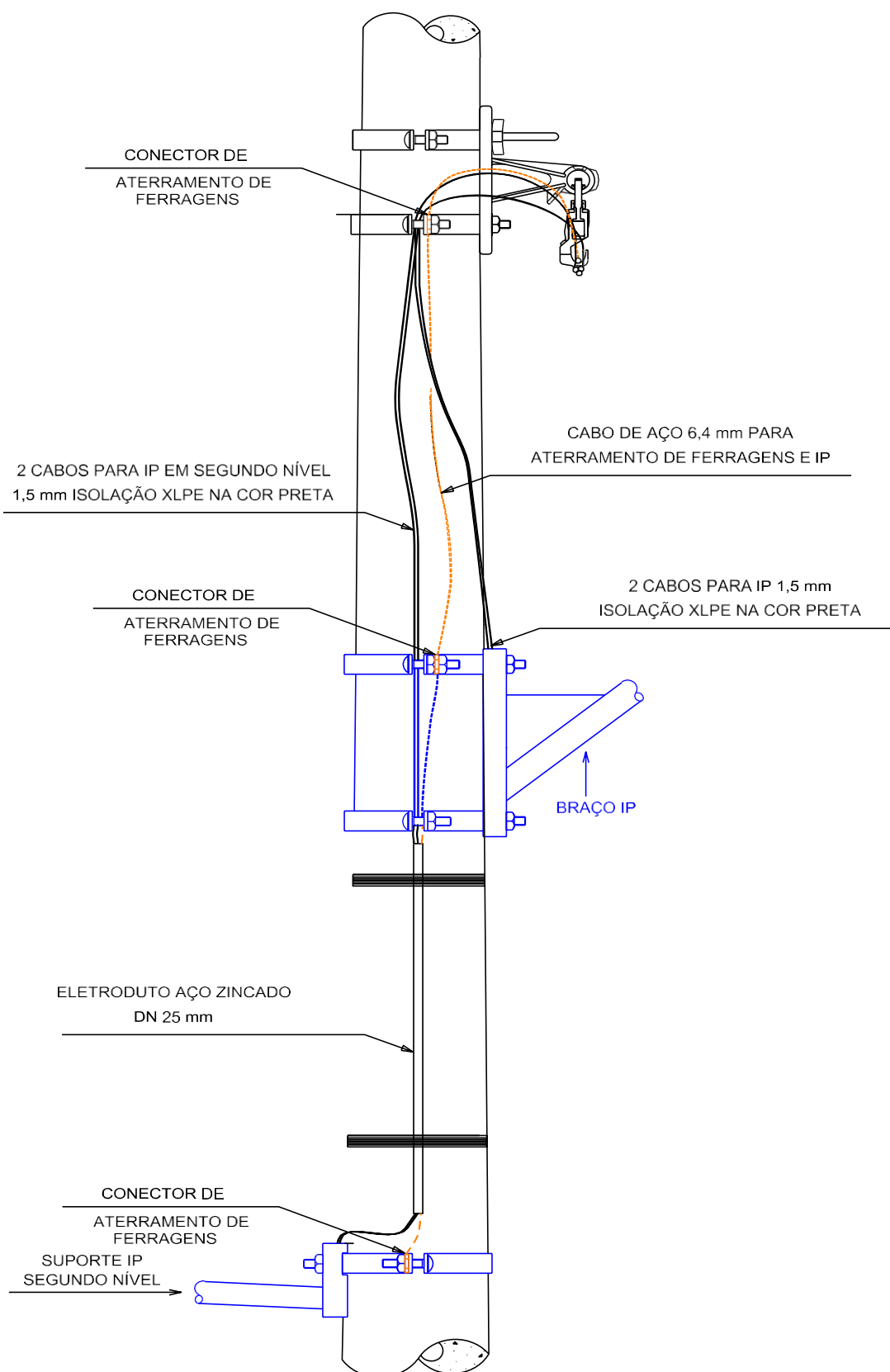
Figura 3 - Aterramento Definitivo de Ferragens e Conexão de Equipamentos de IP em Segundo Nível
