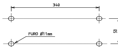
DETALHE DE FURAÇÃO DO BTX
