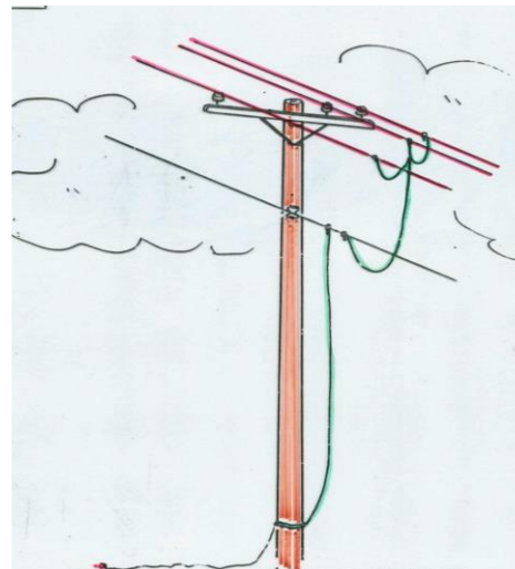
Figura 2: Aterramento em RDR
