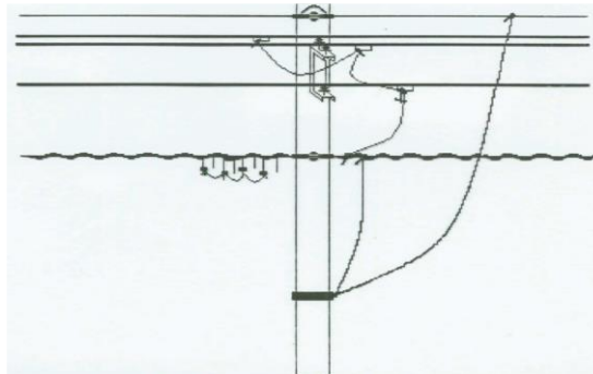
Figura 6: Aterramento em Rede Compacta e Rede Secundária Isolada
