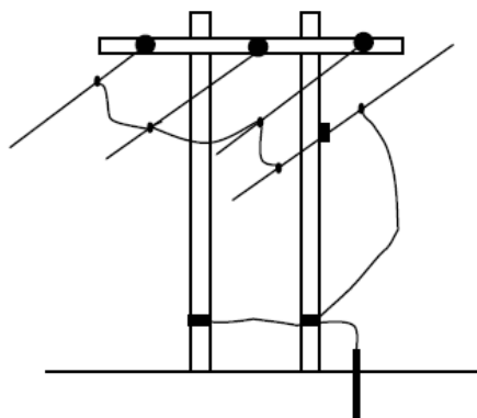
Figura 7: Aterramento em HT
