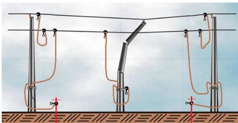
Figura 3: Aterramento em adjacências
