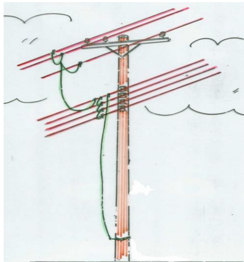
Figura 1: Aterramento de RDU
