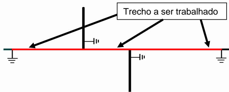
Figura 5: Aterramento em pontos onde há mais de duas possibilidades de alimentação
