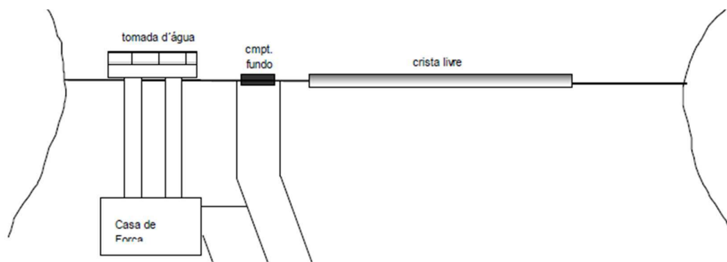
Figura 1 - Estruturas do Empreendimento da PCH Dona Rita
