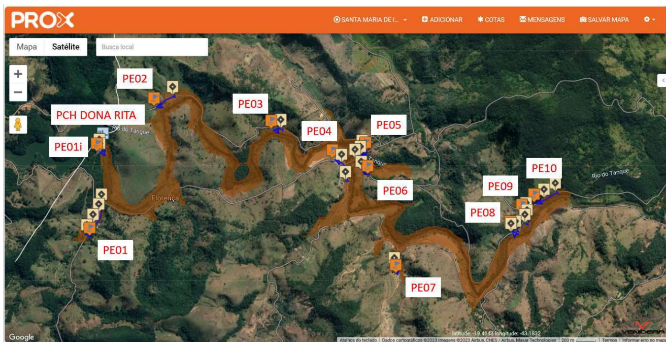
Figura 10 – Localização das placas de sinalização de alerta das Rotas de Fuga e Pontos de Encontro no PROX.
