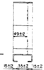
CORTE B-B
