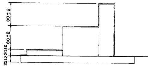
CORTE A-A
